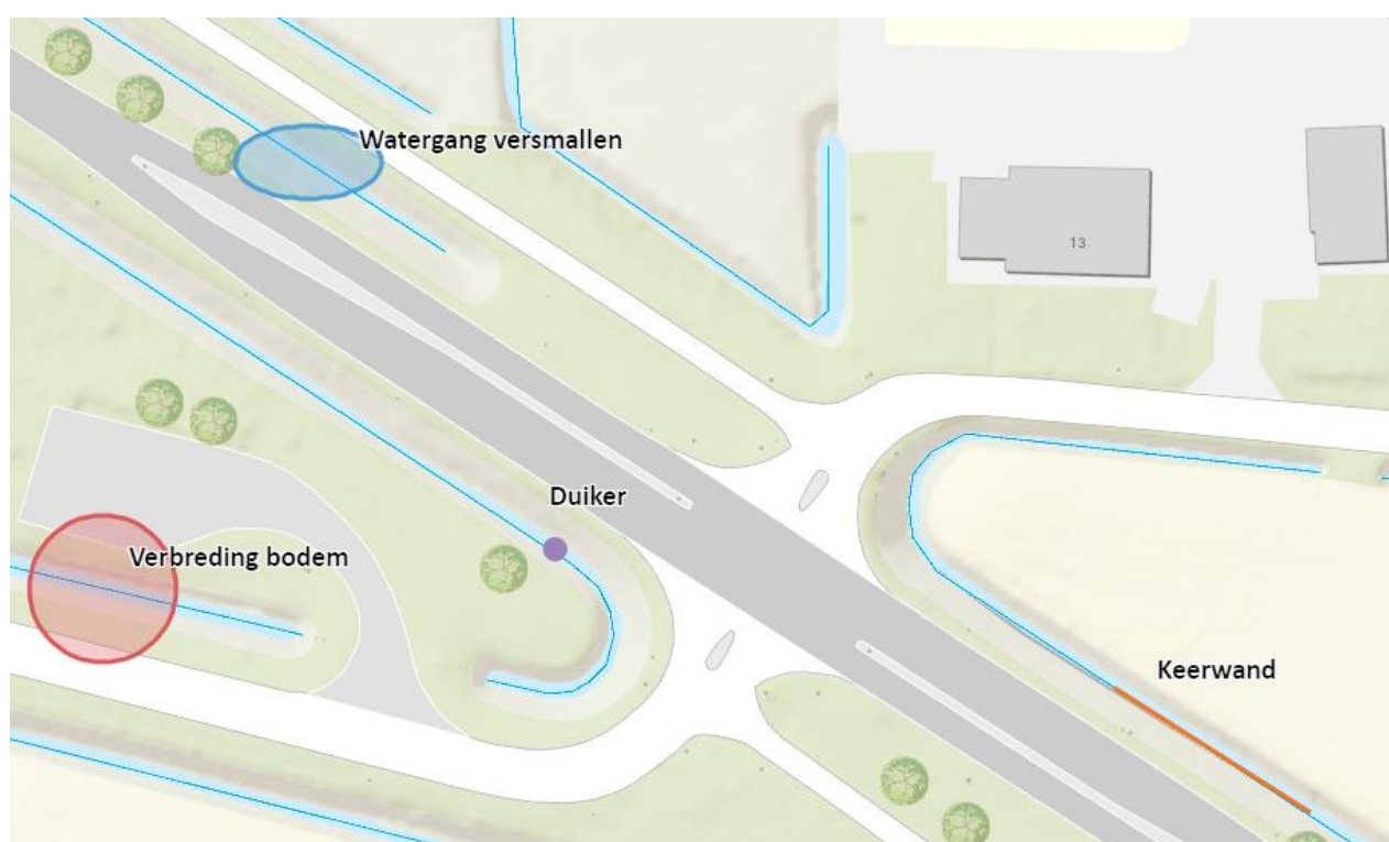
Figuur 1: De paarse stip geeft de locatie van de aan te leggen duiker weer, de oranje lijn geeft de locatie van de aan te leggen keerwand weer, de rode cirkel geeft aan waar de bodem wordt verbreed en de blauwe ellips geeft aan waar de watergang zal worden versmald.
