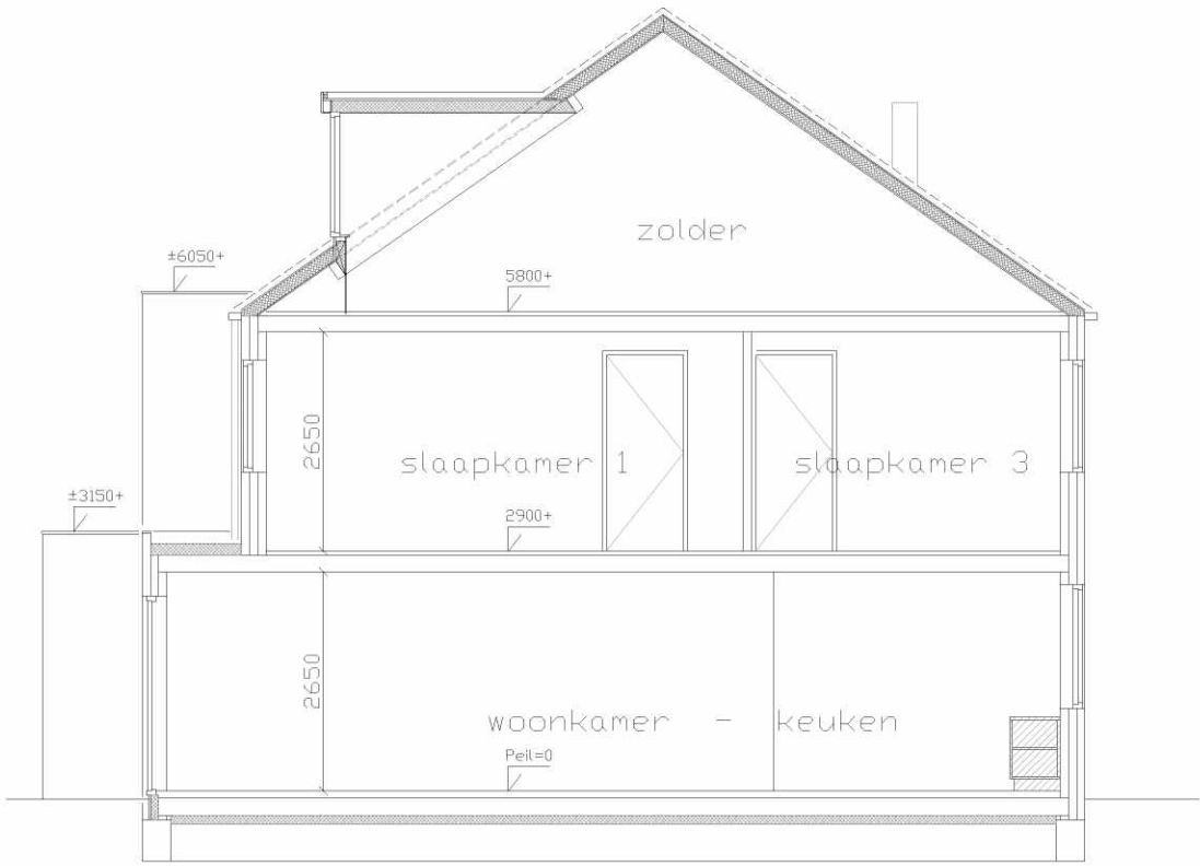
Doorsnede
