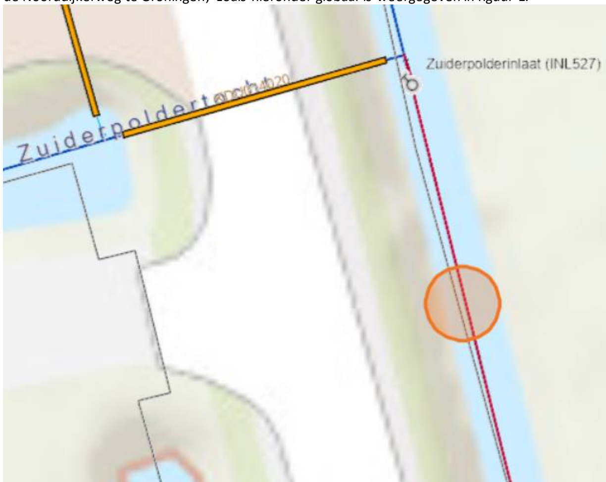
Figuur 1: bestaande duikers en inlaat, de oranje cirkel geeft globaal de locatie van de nieuwe gronddam met inlaatconstructie weer.
