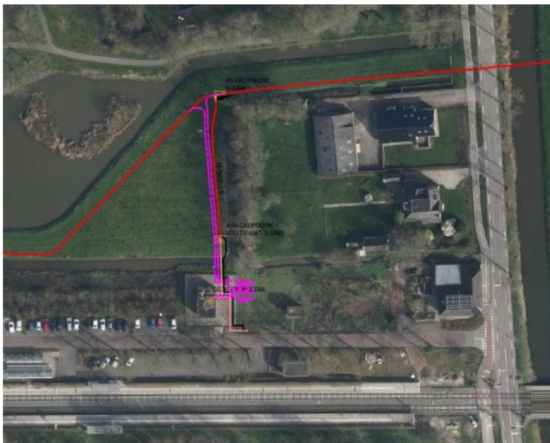
Figuur 1: Overzichtstekening van de werkzaamheden. De rode lijnen zijn de nieuw aan te leggen leidingen.
