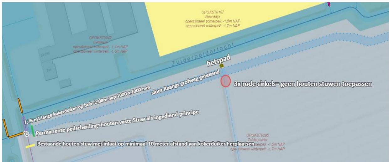
Figuur 2: Aansluiting Noorddijkerweg deel I, conform aanpassing aanvraag d.d. 17 februari 2025.
