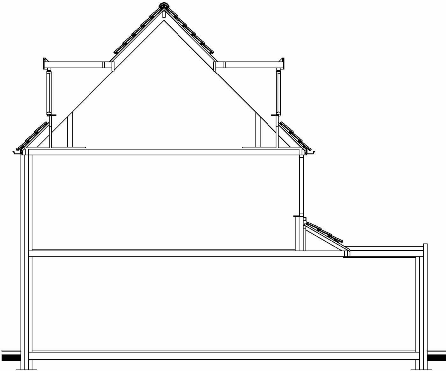
= Doorsnede bestaand =
