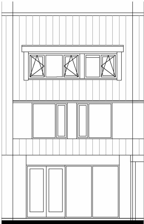
= Achtergevel bestaand =
