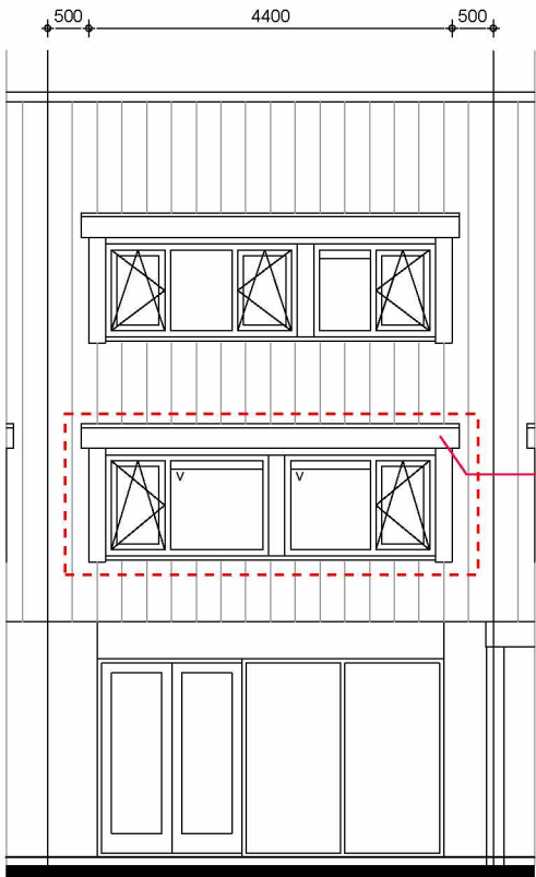
= Achtergevel nieuw =
