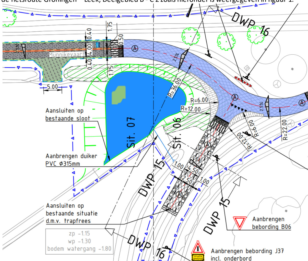
Figuur 1: situatietekening van de te graven waterpartij.
