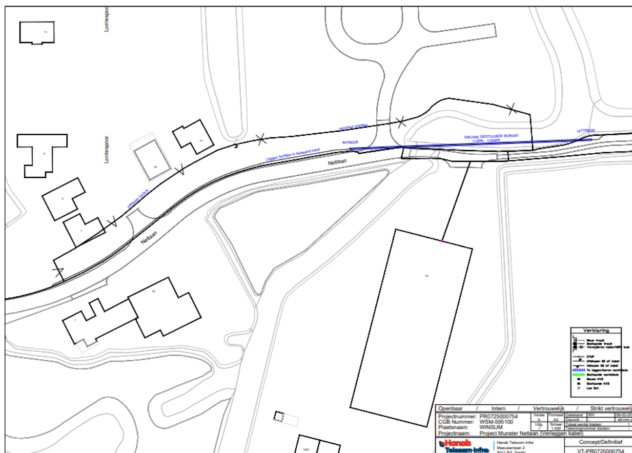
Figuur 1: Overzichtstekening van de werkzaamheden. De blauwe lijn geeft de locatie weer van de te maken boring.
