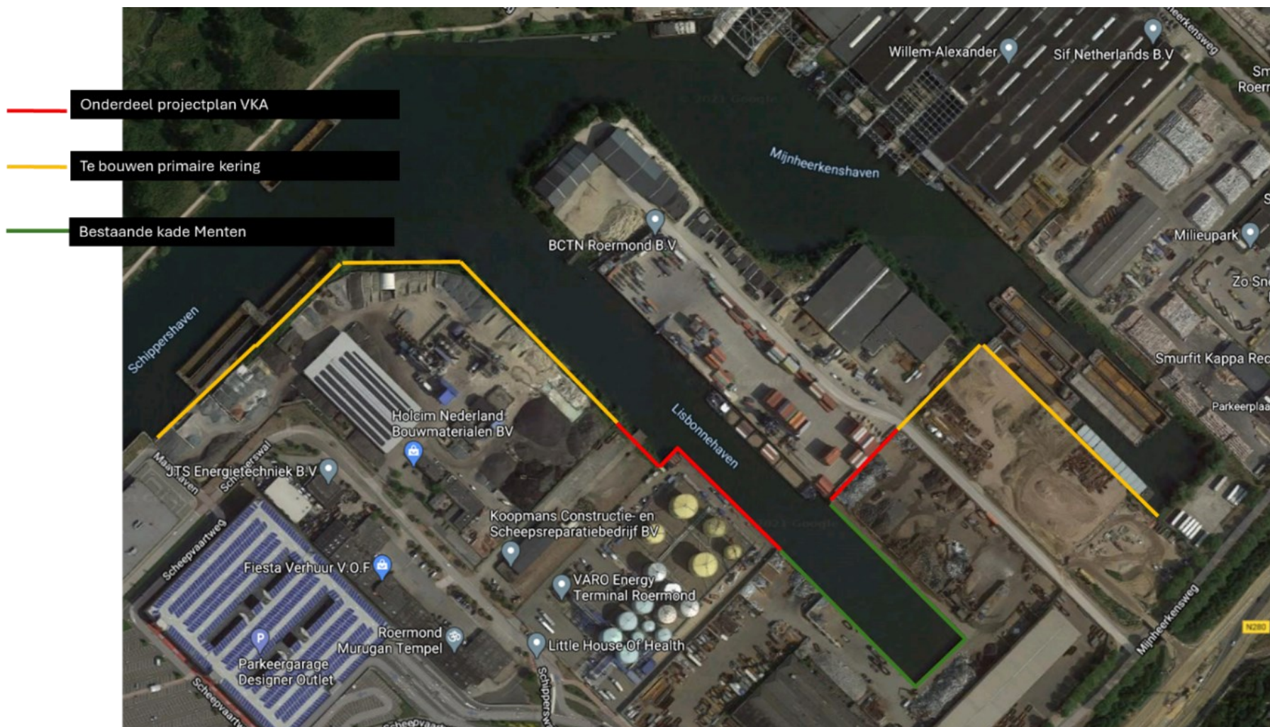
Figuur 2: Voorkeursscenario primaire keringen (gele lijn) Port of Roermond (groene lijn is bestaand)
