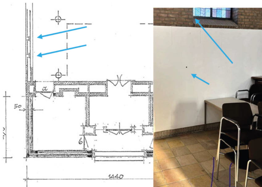
Links Knipsel van tekening 'nieuwe frontbouw W251 BLv1 d.d. 18-06-1959. Rechts foto met boorgat en kozijn aangeven.
