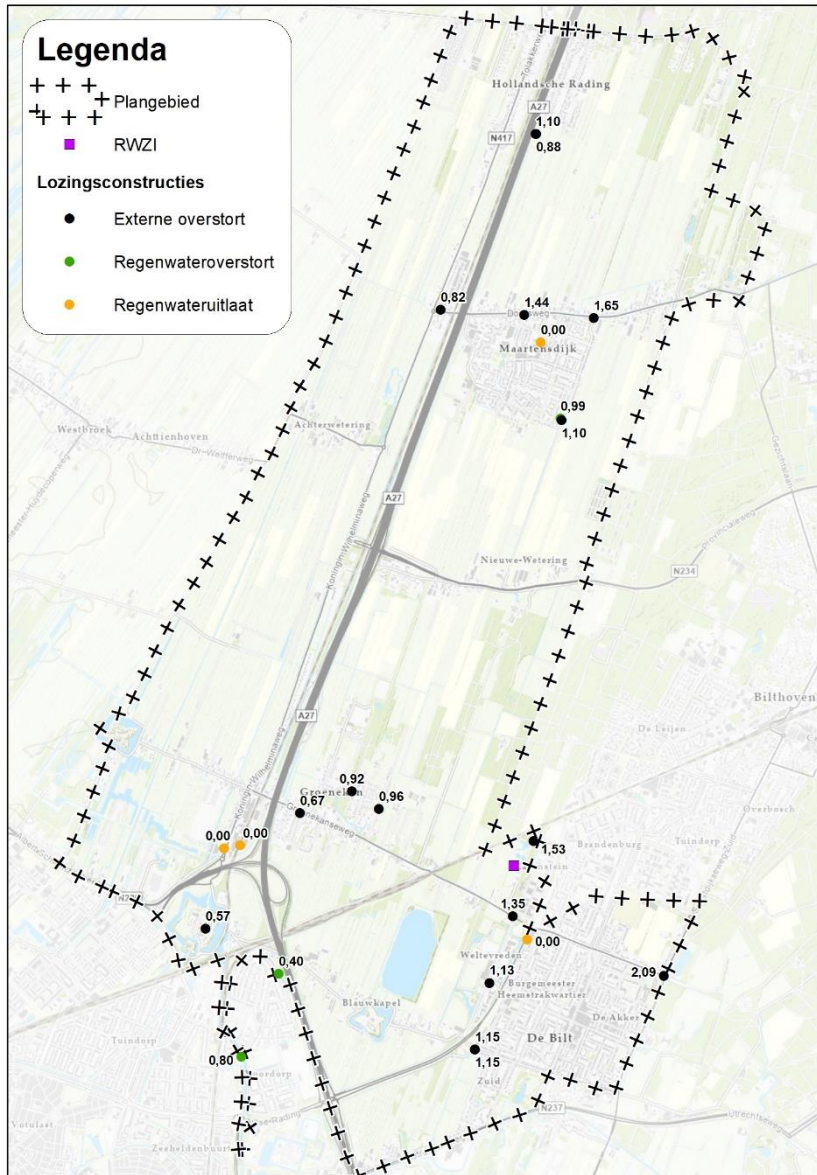
Figuur 9 Locaties lozingsconstructies en rioolwaterzuiveringsinstallatie (RWZI) De Bilt. De cijfers geven de hoogte van de overstordrempels aan in m t.o.v. NAP
