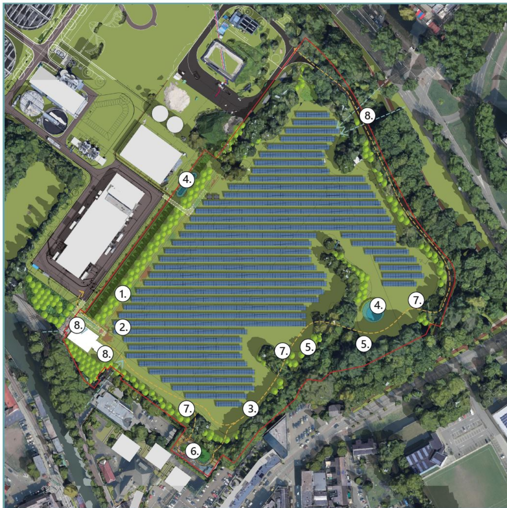
afb. 17: structuurschets inrichting zonneweide RWZI met referentiebeelden ( www.haverdroeze.nl )
