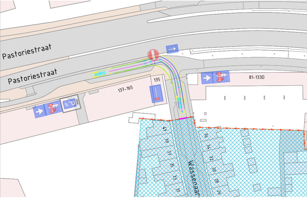
Rijcurves Inrit vanaf Pastoriestraat (Vrachtwagen 12m)
