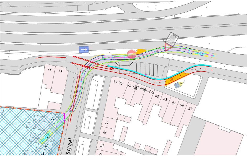
Rijcurves Inrit vanaf Verwerstraat (Trekker oplegger)
