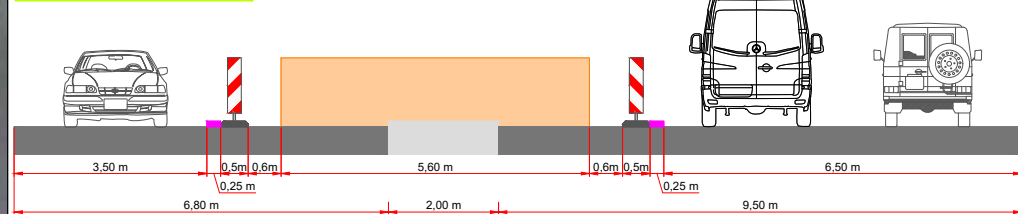
Dwarsdoorsnede A-A
