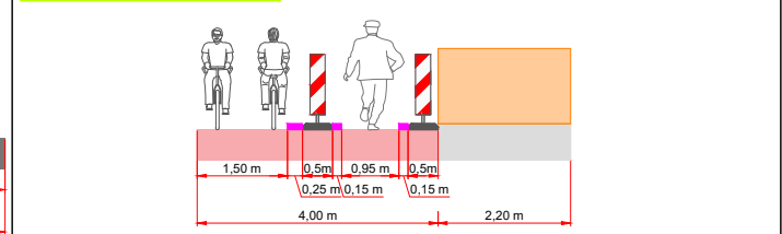
Dwarsdoorsnede B-B
