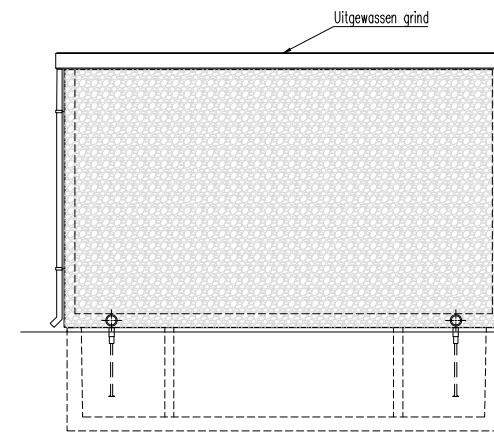
Aanzicht C
