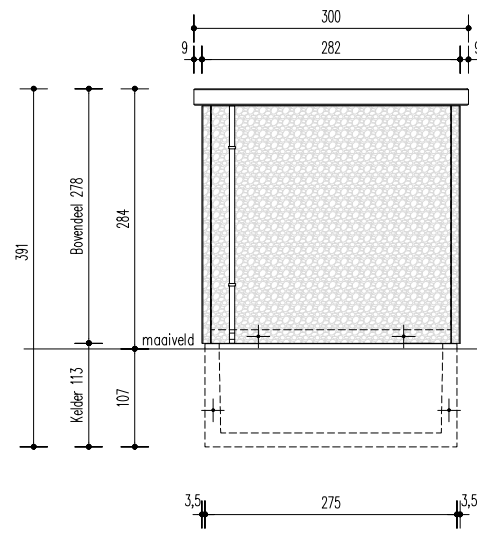
Aanzicht B
