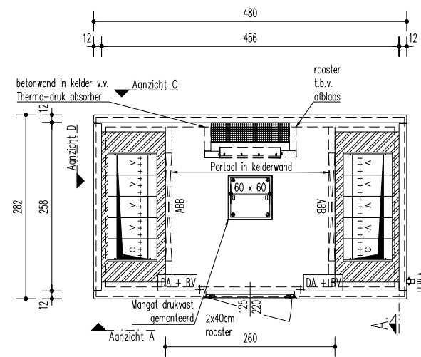
Plattegrond
