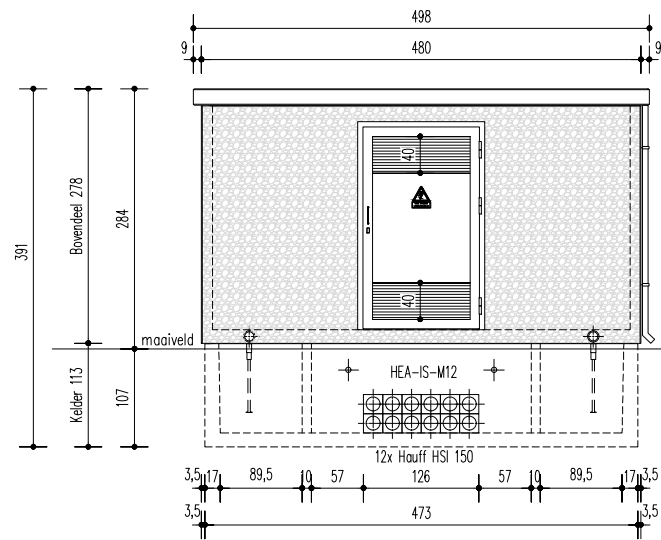
Aanzicht A
