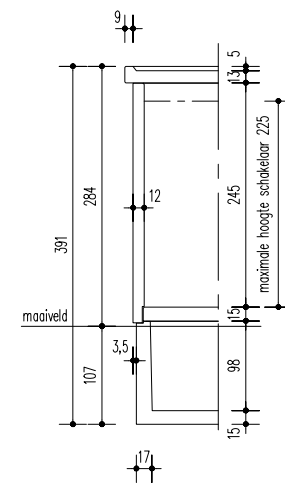
Doorsnede A. Station met vaste kelder
