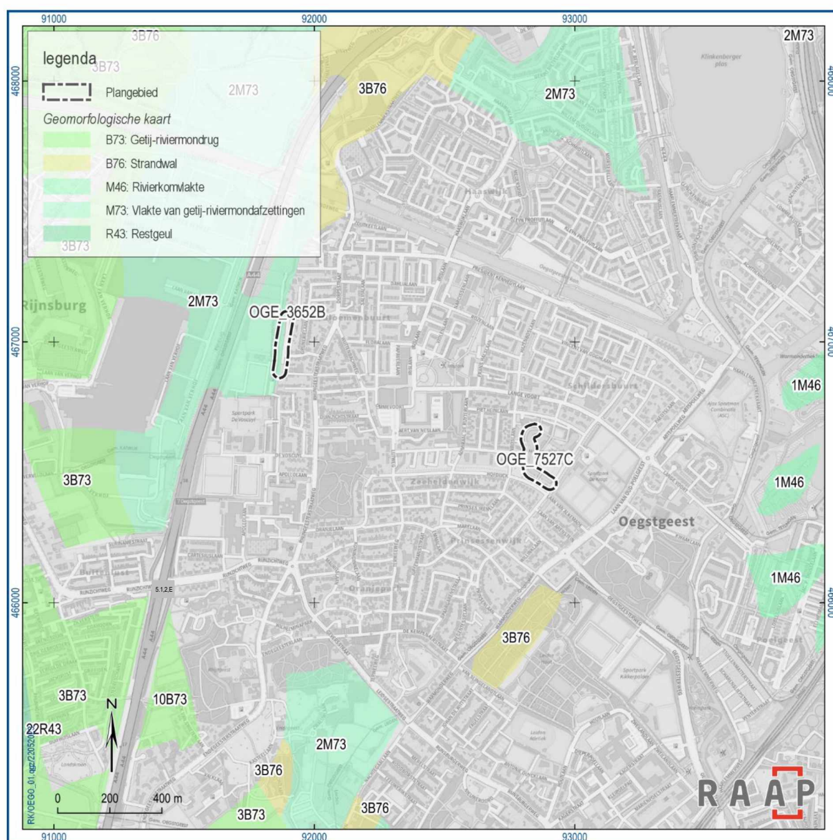
Figuur 7. Geomorfologie.
