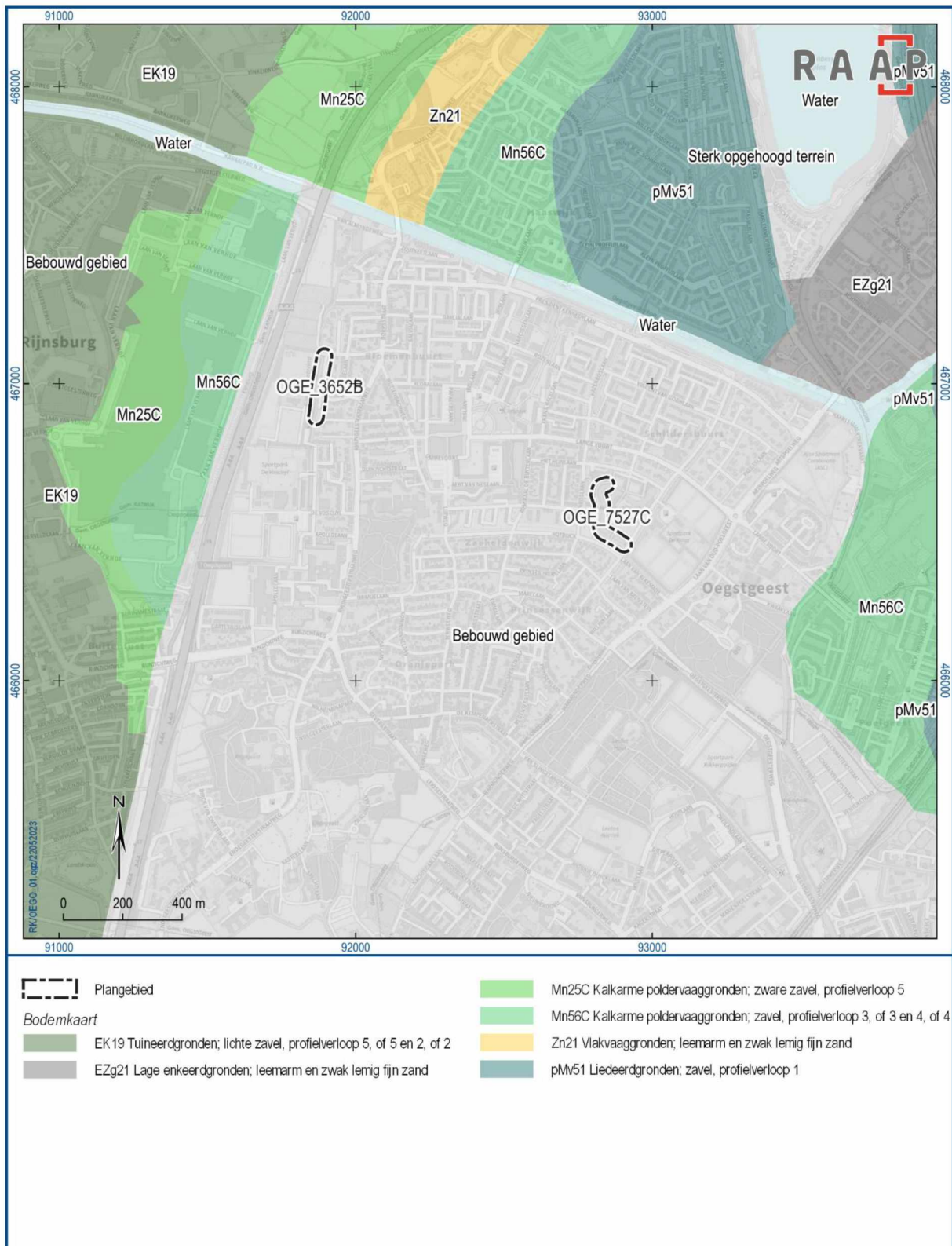
Figuur 9. Bodemkaart.
