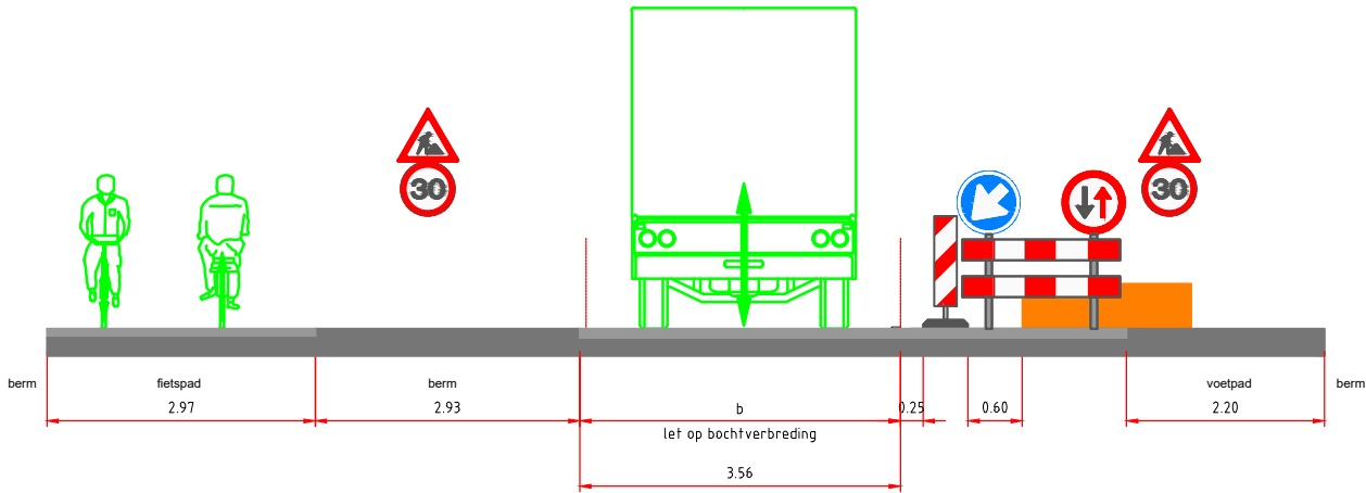
Doorsnede A-A
