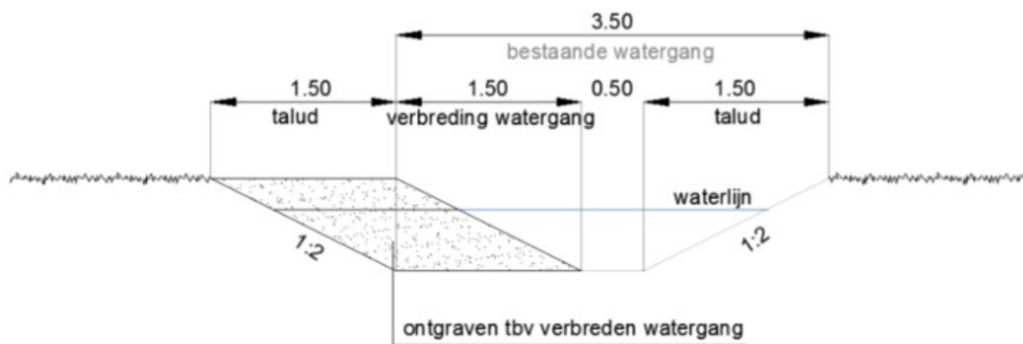
Figuur 7: Principeprofiel verruiming bestaande greppel binnenterrein testbaan
