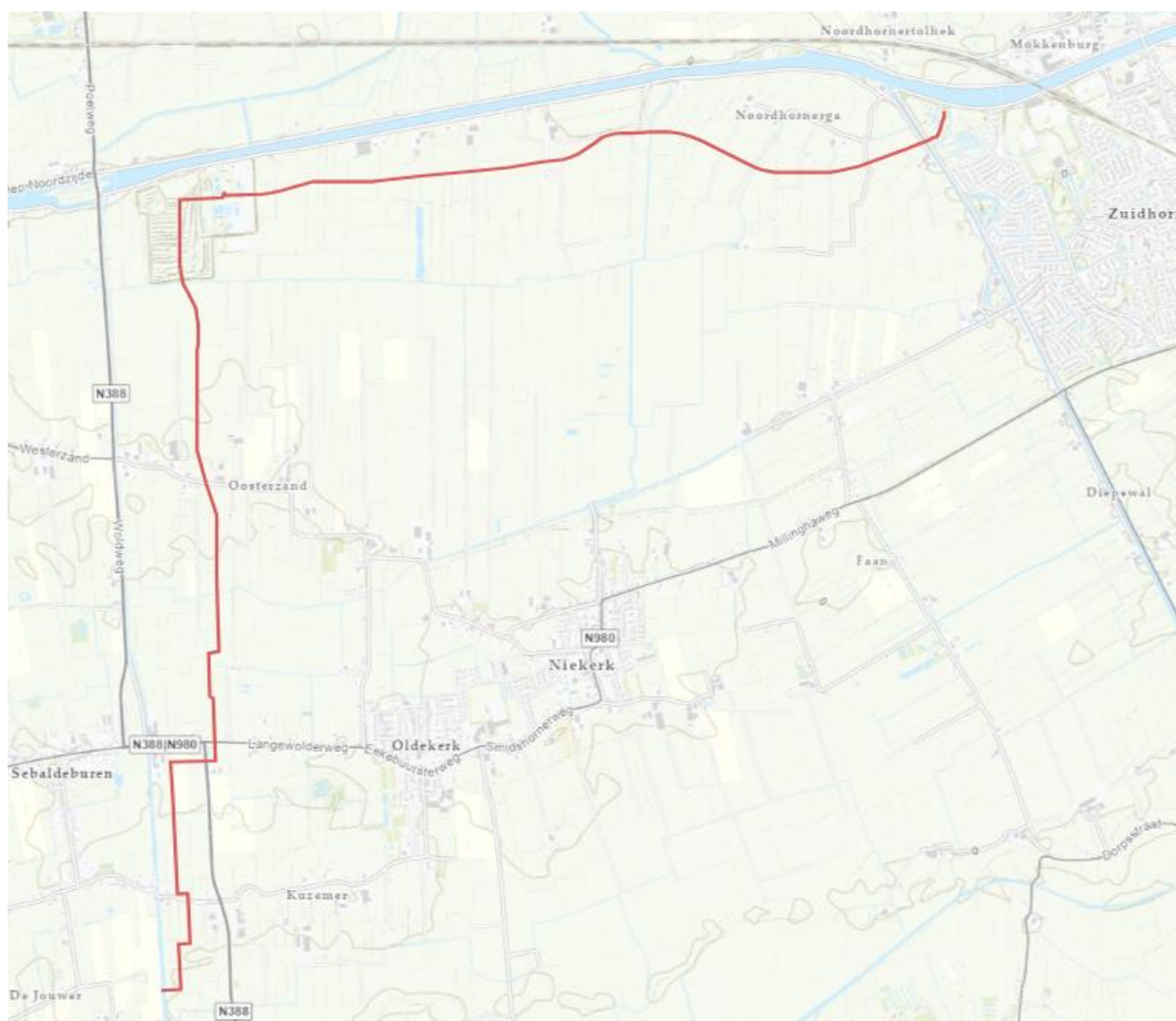
Figuur 1: In het rood de aan te leggen leidingtracés
