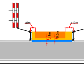
Werkvakindeling ETW
