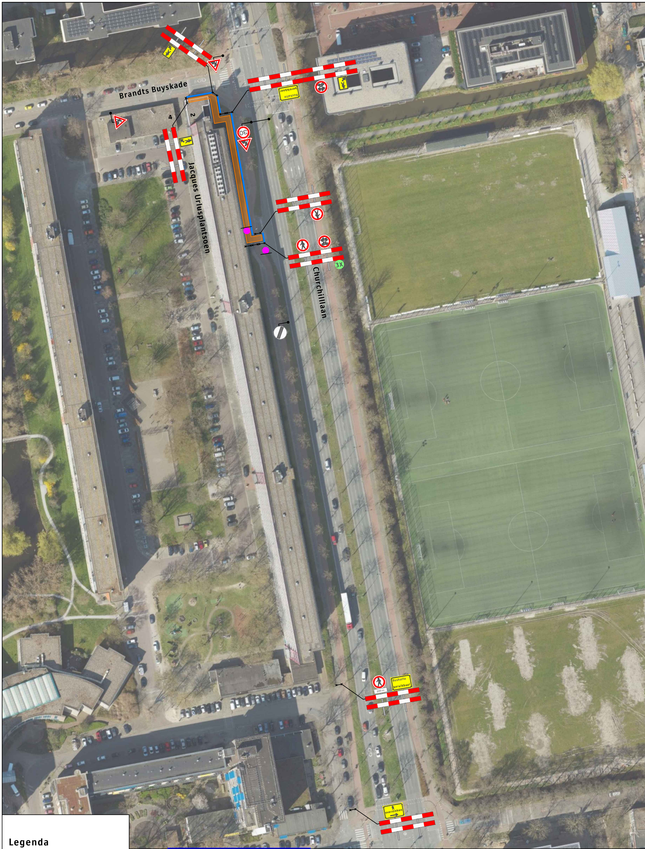
Werkvakindeling voetpad
