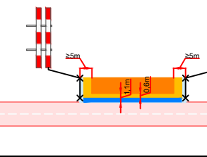
Werkvakindeling fietspad
