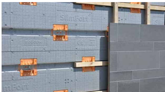
Afwerking met tegels
