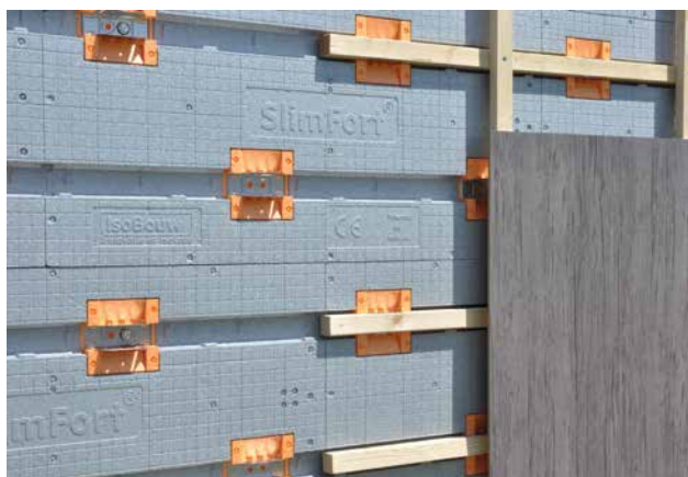
Afwerking met geperste minerale wol platen
