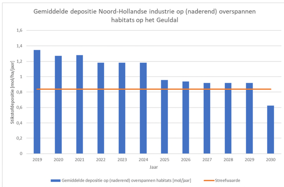
Figuur B3-5: Toekomstige ontwikkeling stikstofdepositie Geuldal
