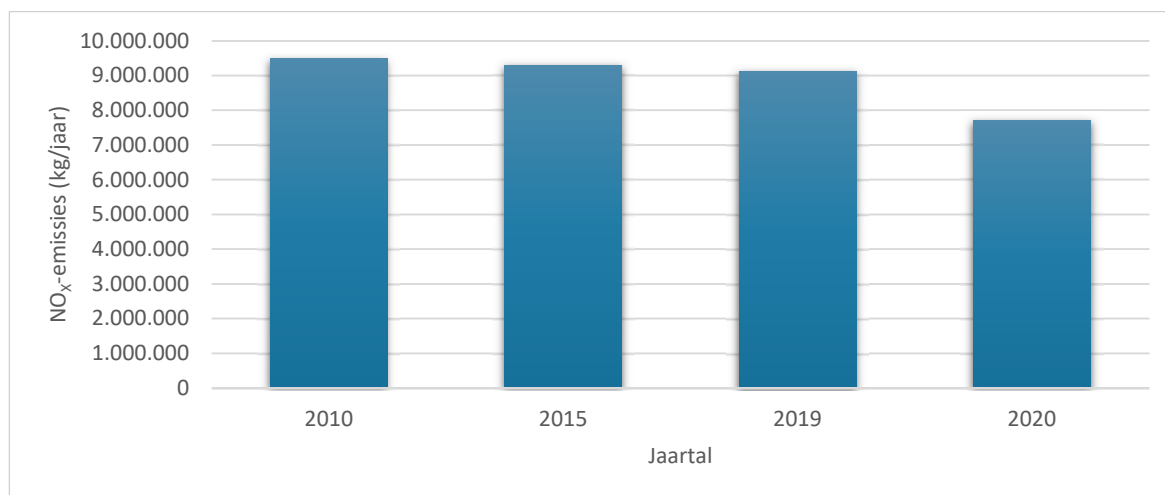
Figuur 5-1: Historische ontwikkeling NO x -emissies (kg/jaar)
