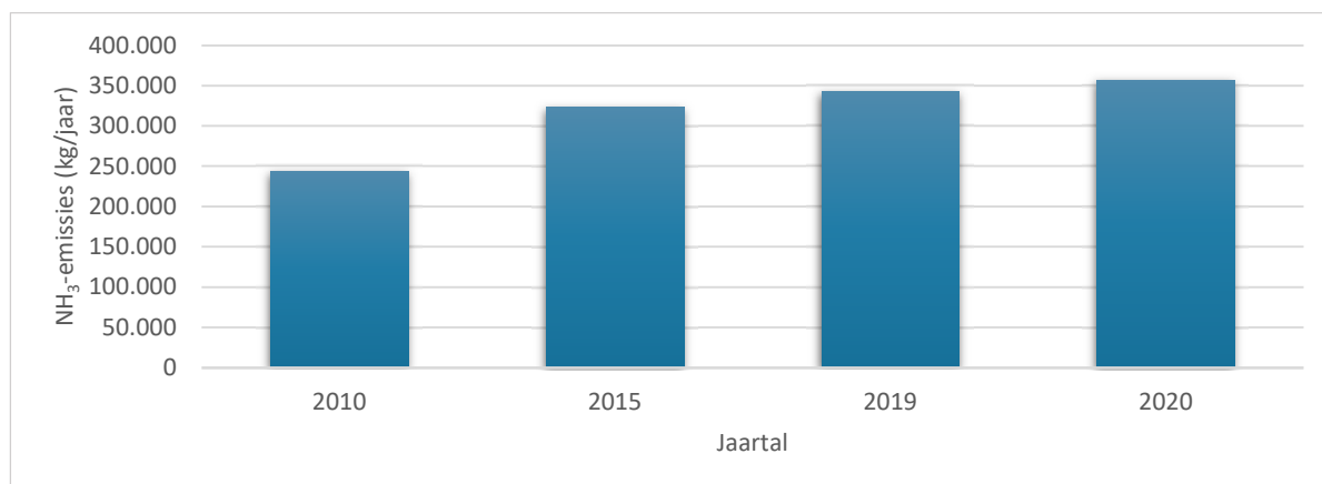
Figuur 5-2: Historische ontwikkeling NH 3 -emissies (kg/jaar)
