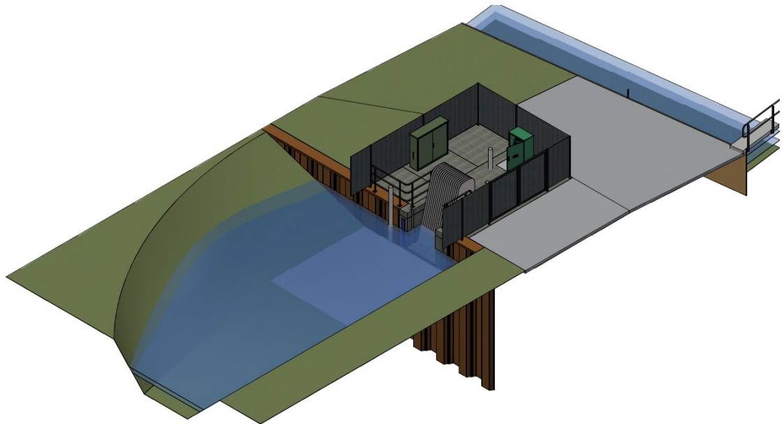
Figuur 2. 3D ontwerp gemaal Emsterbroek inclusief de nieuwe damwand en bestaande brug (bron Waterschap Vallei en Veluwe).
