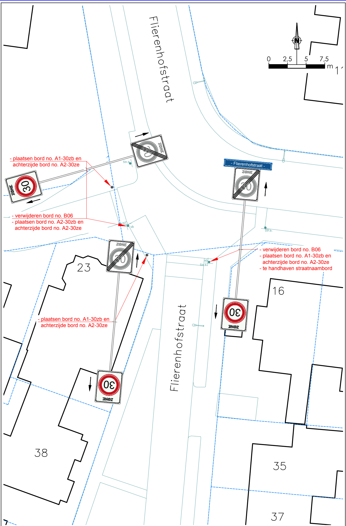
2. Anpassing t.b.v. 30 km/h zone -- Wardstraat Flierenhofstraat
