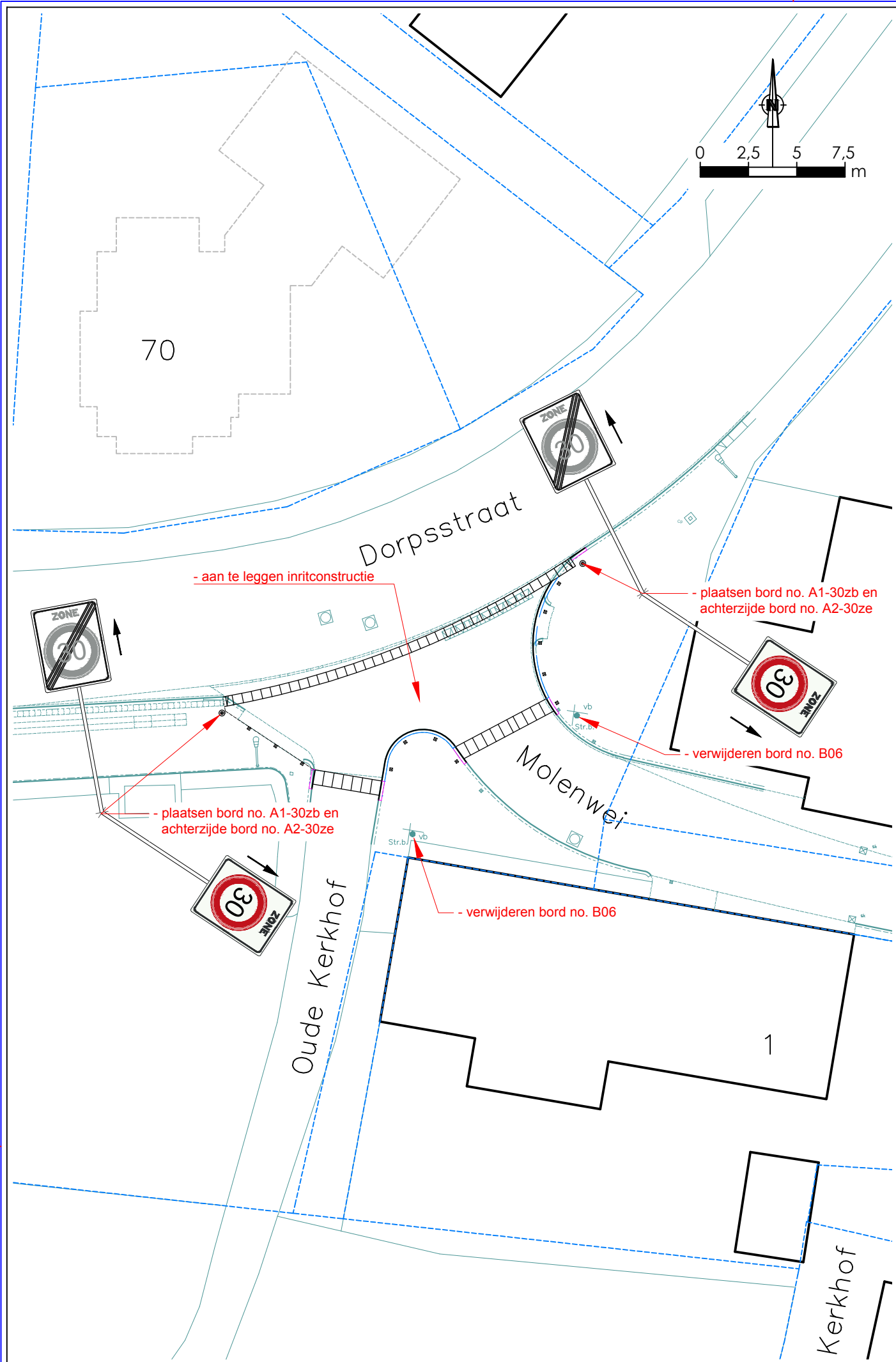
1. Anpassing t.b.v. 30 km/h zone - Dorpsstraat - Molenweg
