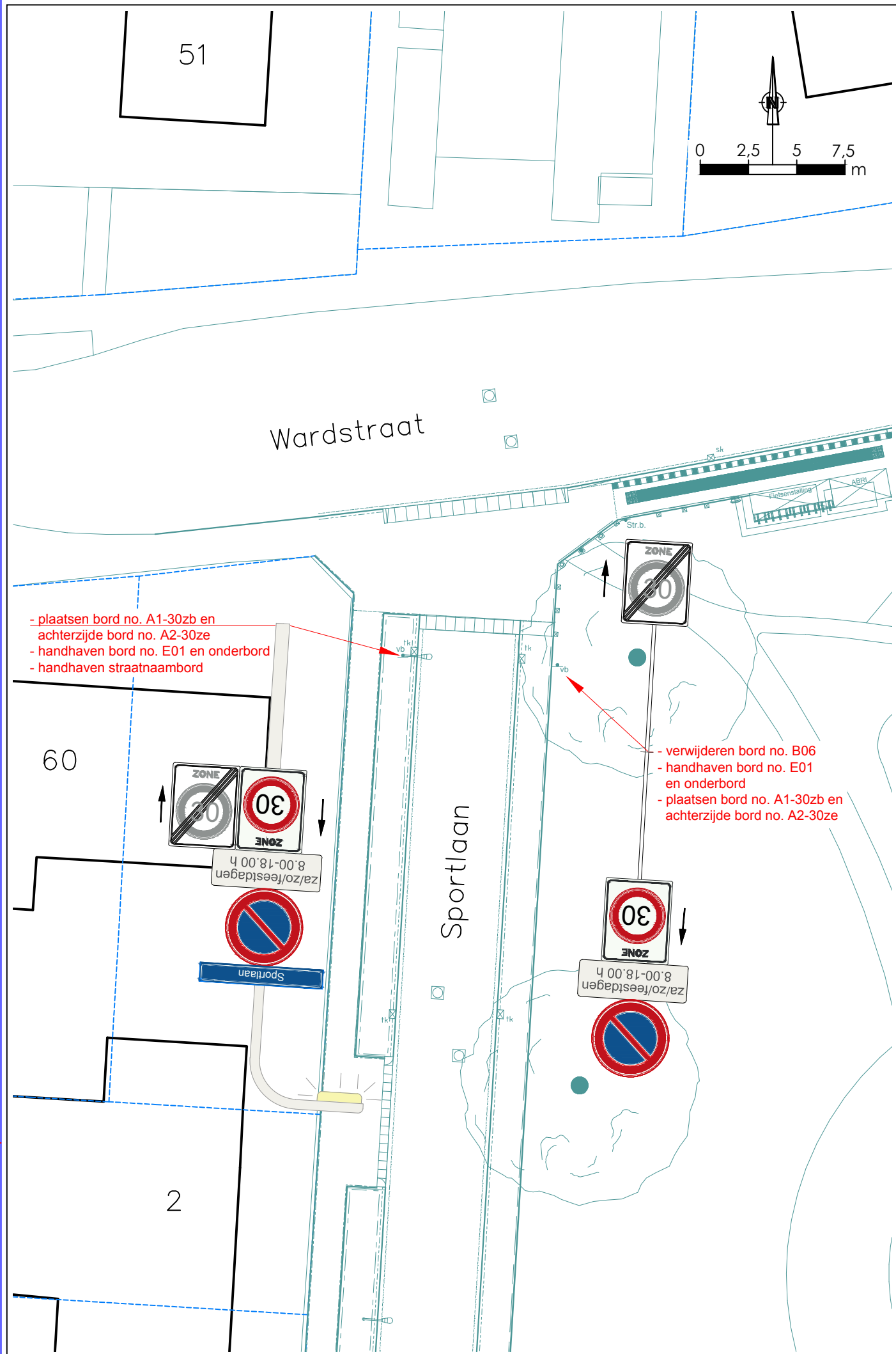
4. Anpassing t.b.v. 30 km/h zone -- Wardstraat - Sportlaan
