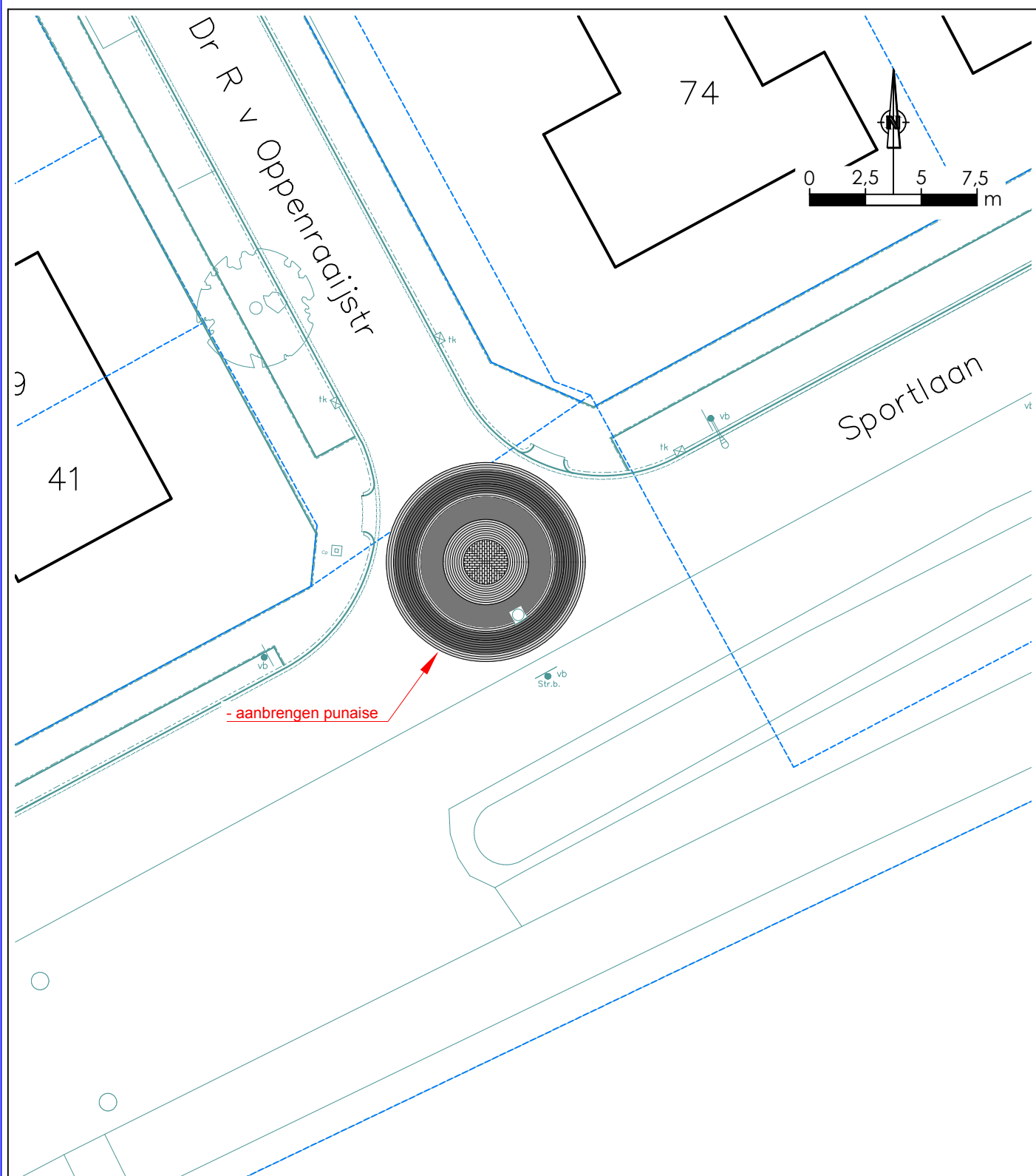
7. Anpassing t.b.v. 30 km/h zone -- Dr. R v Oppenraaijstraat - Sportlaan
