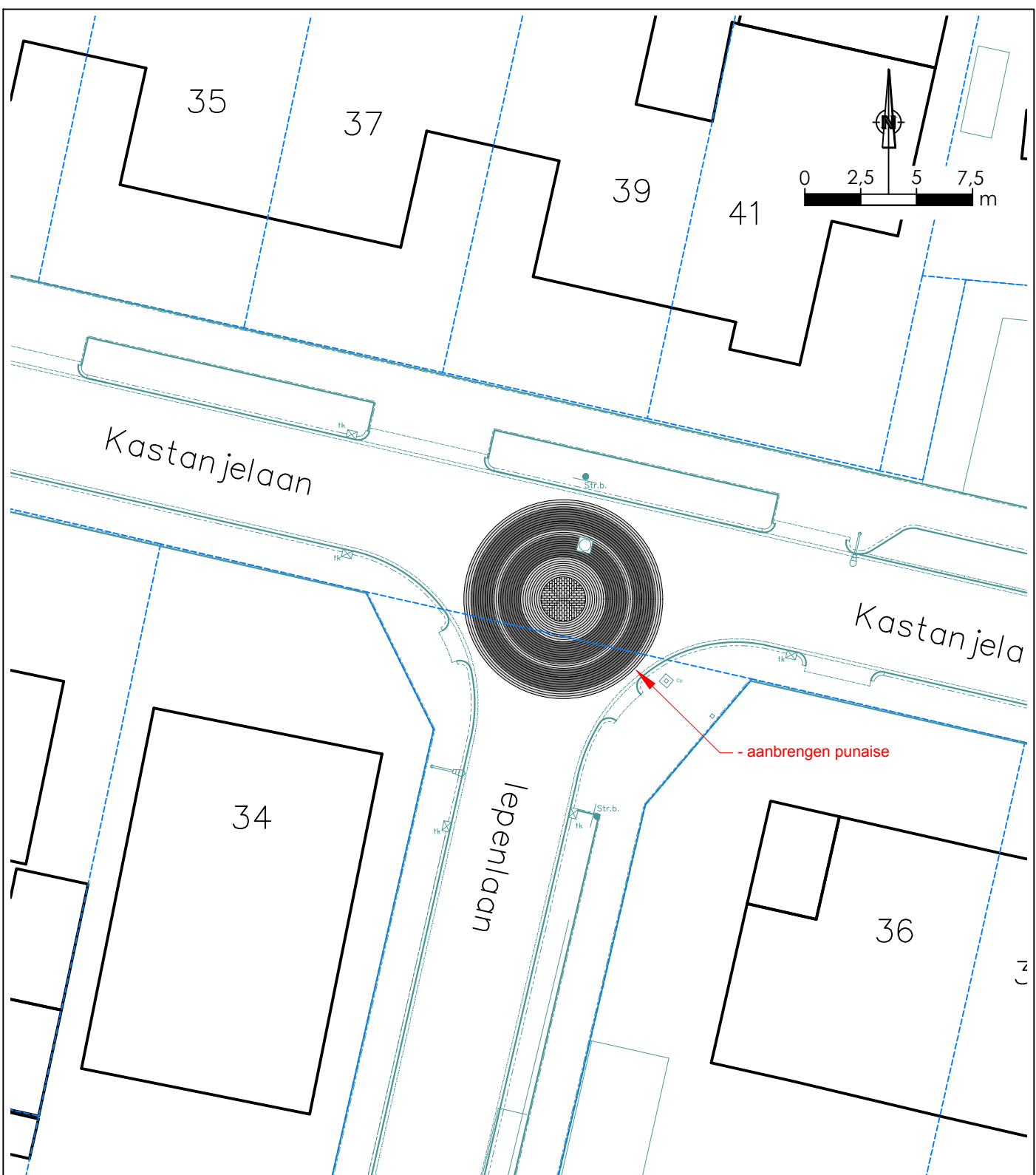
8. Anpassing t.b.v. 30 km/h zone -- Kastanjelaan - Iepenlaan
