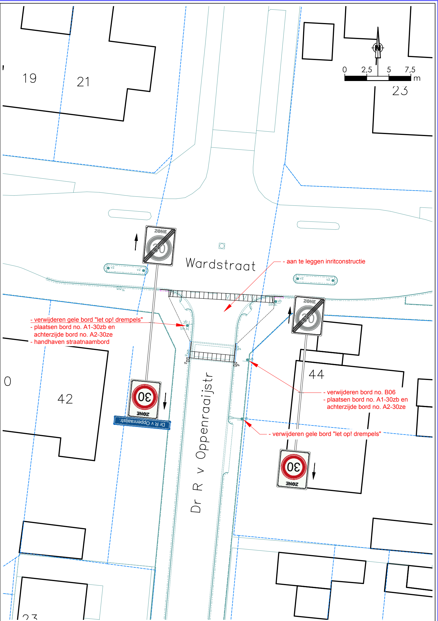
3. Anpassing t.b.v. 30 km/h zone -- Wardstraat Dr.R v Oppenraaijstraat
