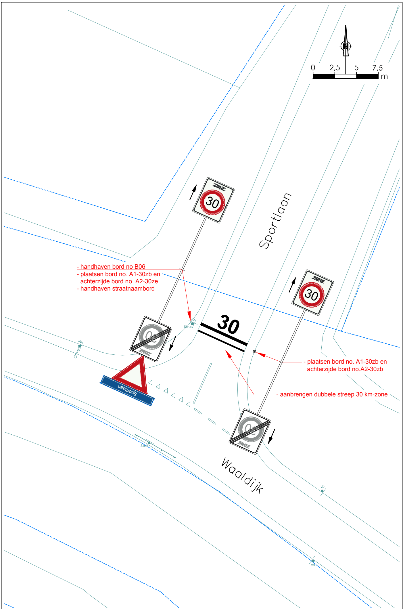
5. Anpassing t.b.v. 30 km/h zone -- Sportlaan - Waaldijk
