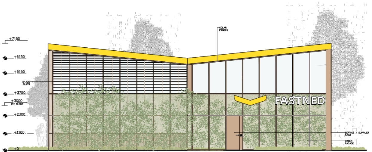
BACK ELEVATION 1:150
