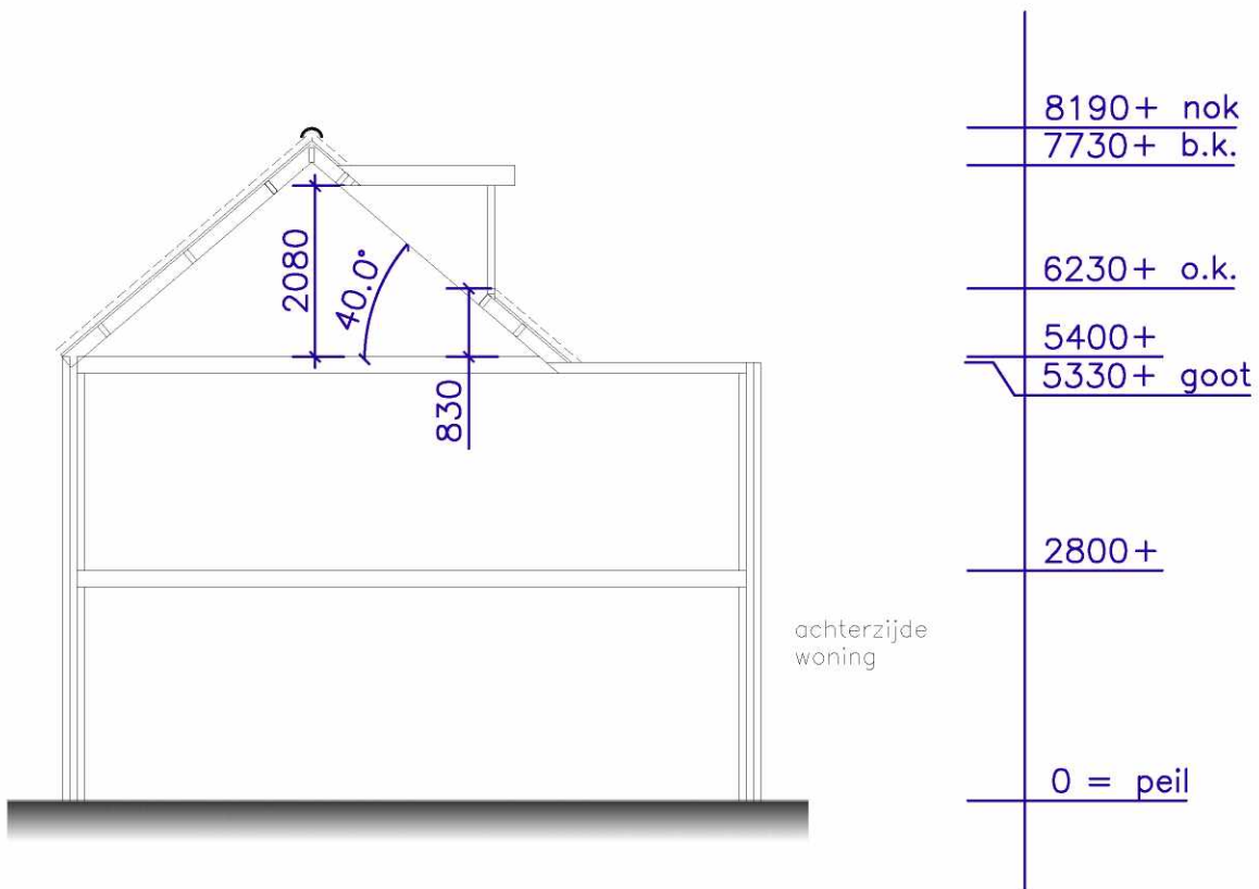
DOORSNEDE NIEUW
