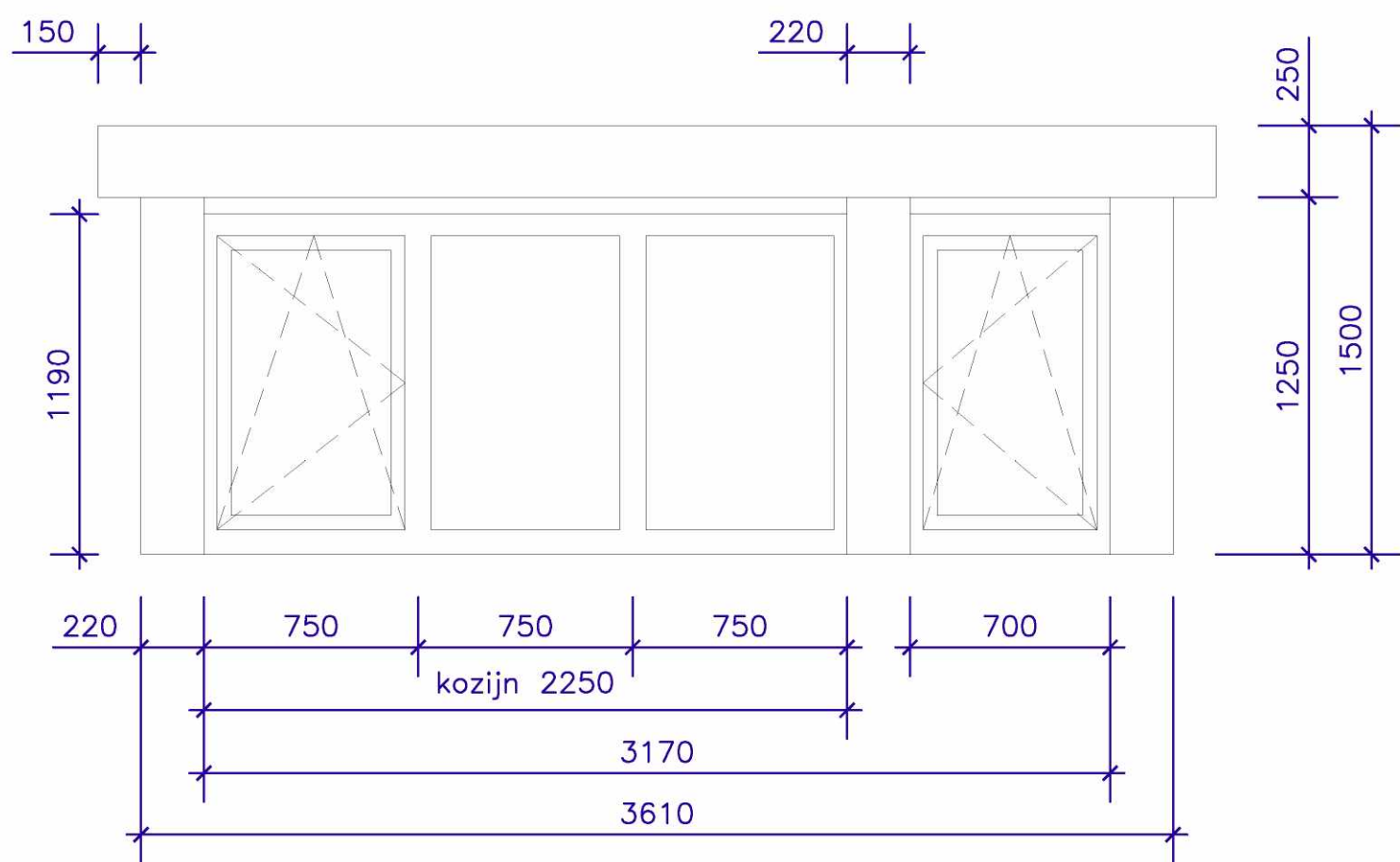
AANZICHT DAKKAPEL ACHTERGEVEL
