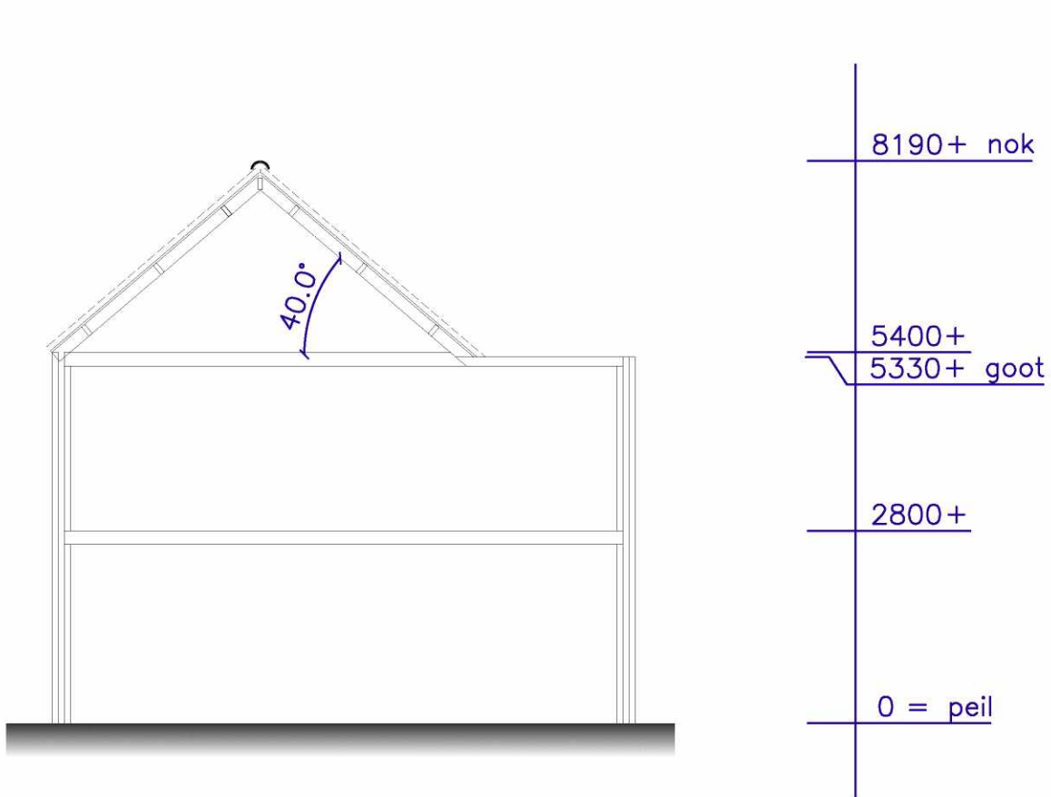
DOORSNEDE BESTAAND
