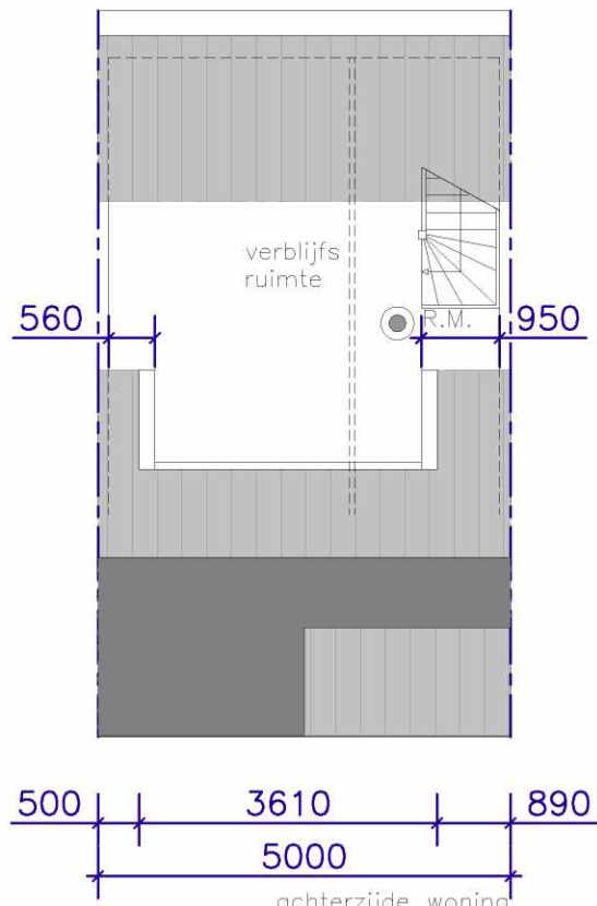
INDELING NIEUW
