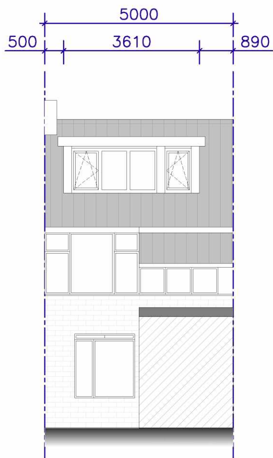
ACHTERGEVEL NIEUW
