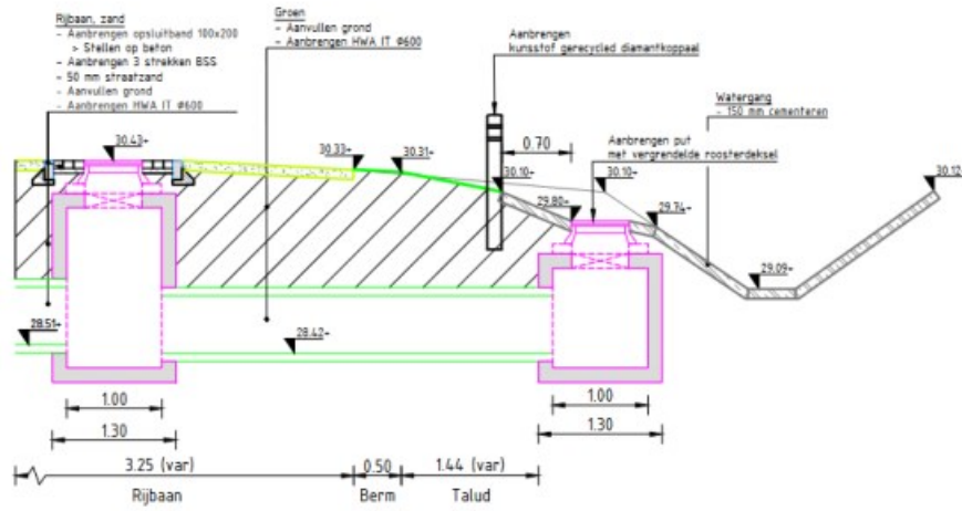
Dwarsprofiel uitstroomvoorziening
