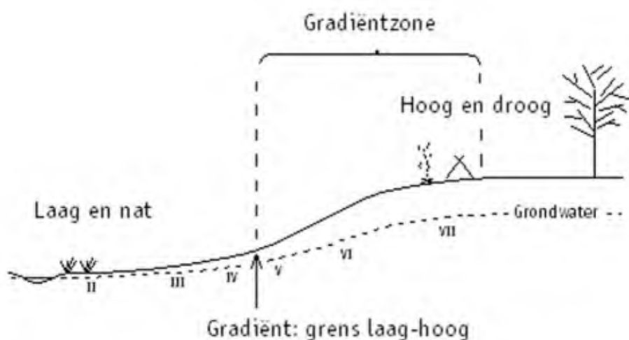
Figuur 15. Gradiëntzones.
