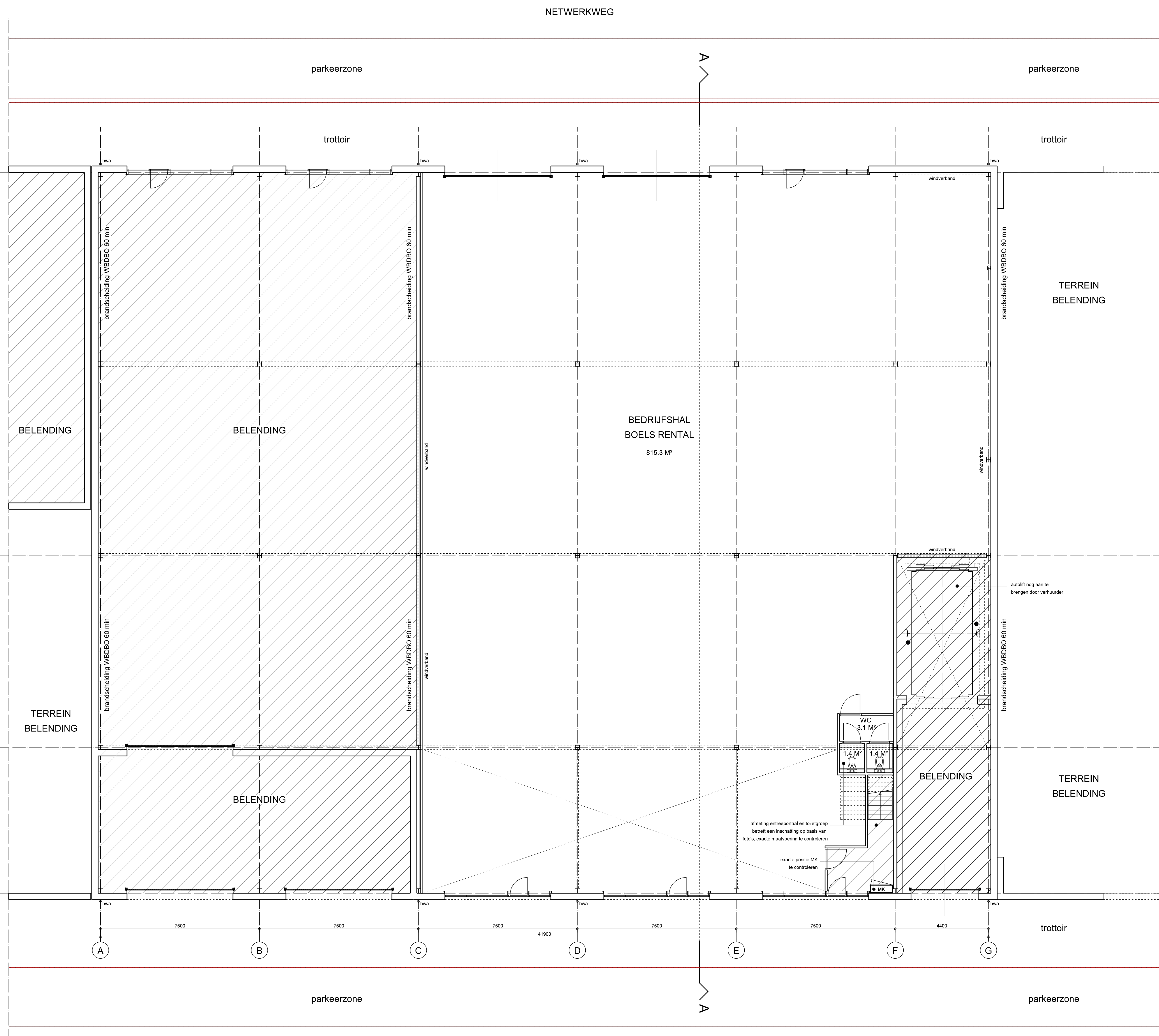
BEGANE GROND
