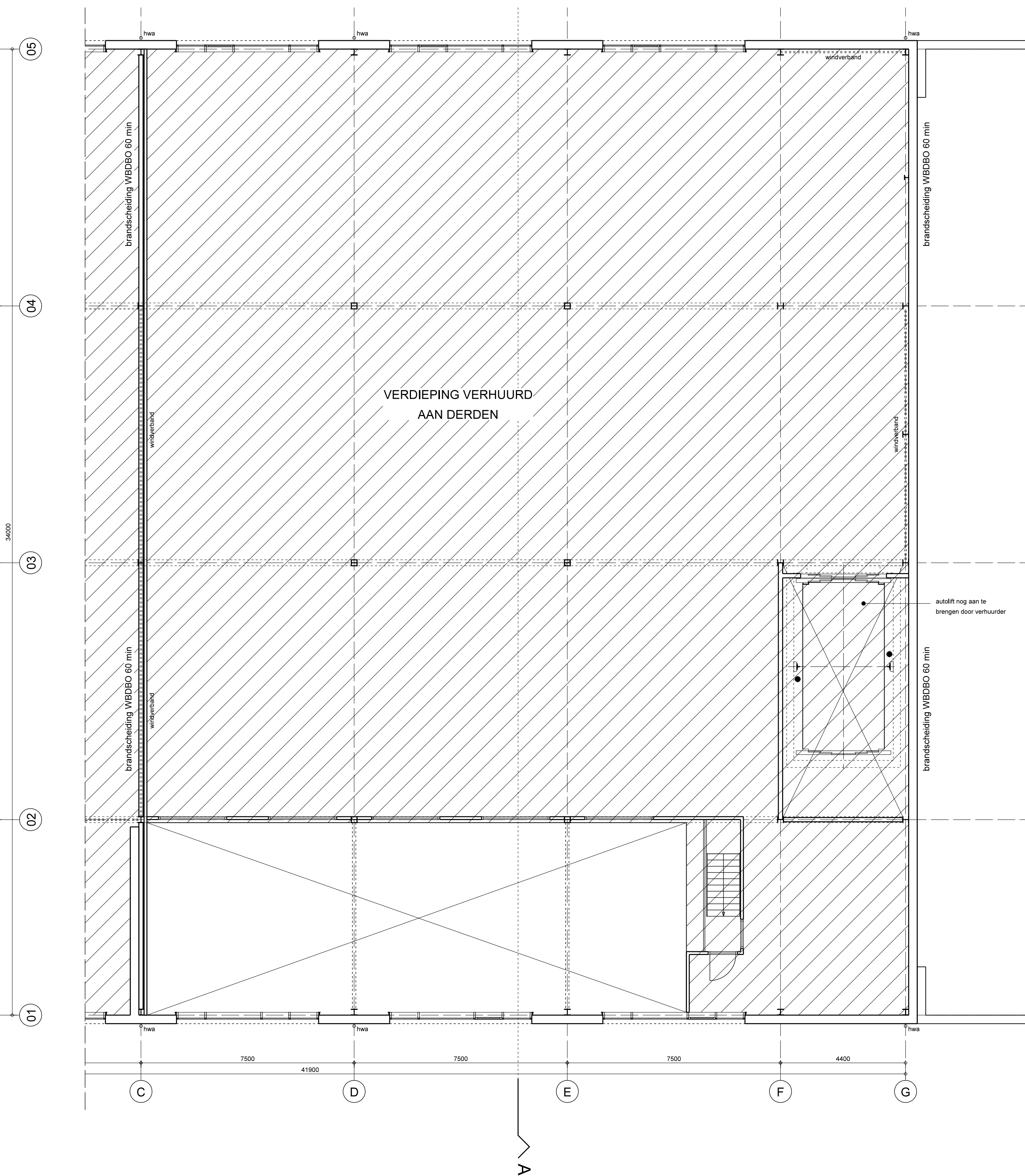
EERSTE VERDIEPING
