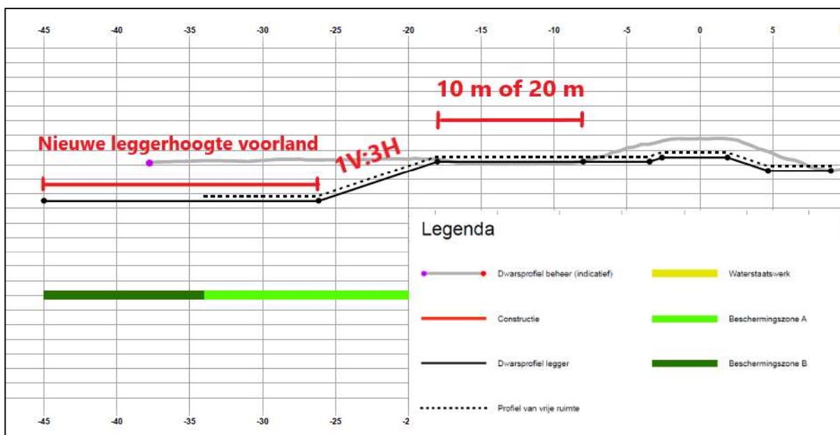
figuur 3-2: dwarsdoorsnede leggerprofiel met hoog voorland
