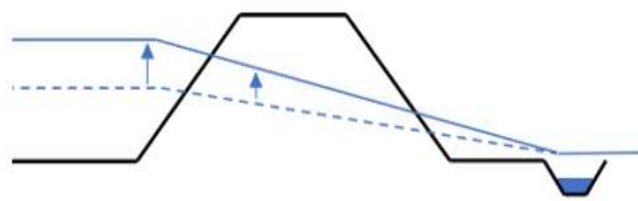
figuur 2-7: actualisatie stijghoogte in watervoerend pakket gegeven opdrijven/opbarsten.
