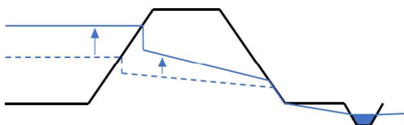
figuur 2-8: actualisatie freatische waterspanningen
