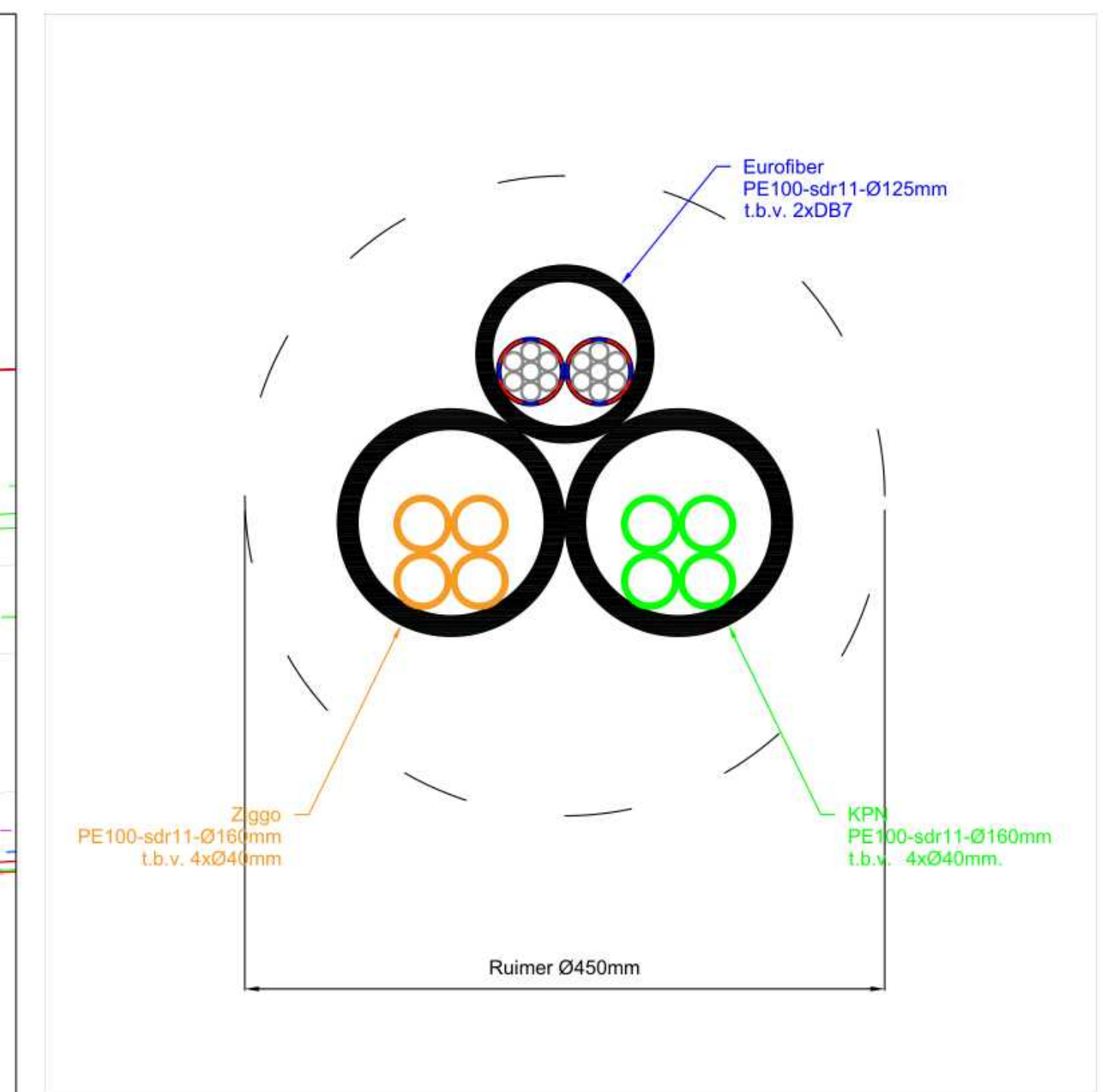
Dwarsdoorsnede buis (schaal 1:4)
