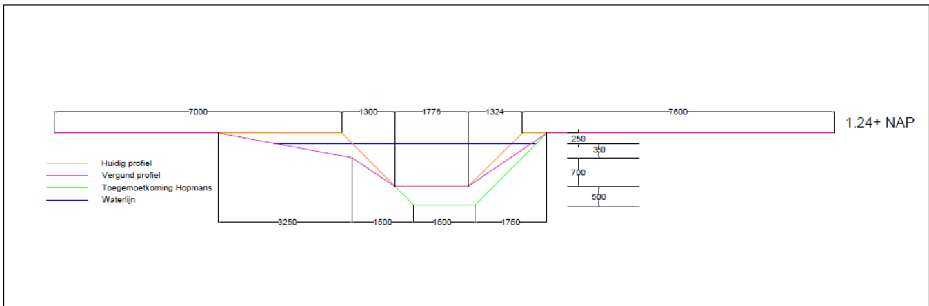
Dwarsprofiel bodem uitdiepen 500mm
