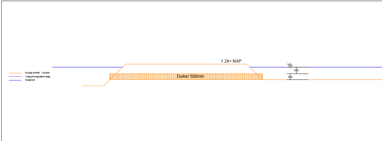
Dwarsprofiel huidige situatie
