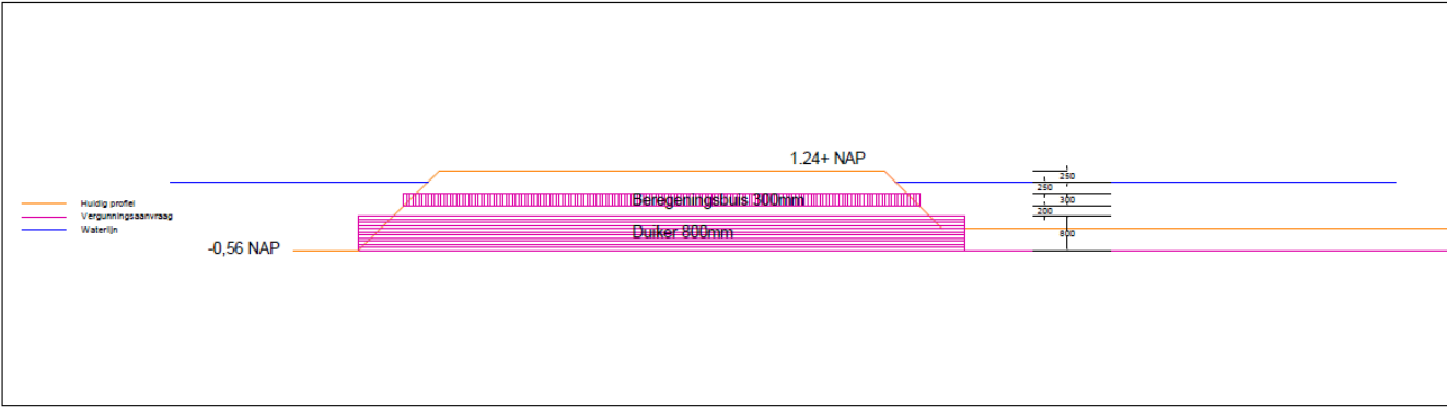
Dwarsprofiel toekomstige situatie
