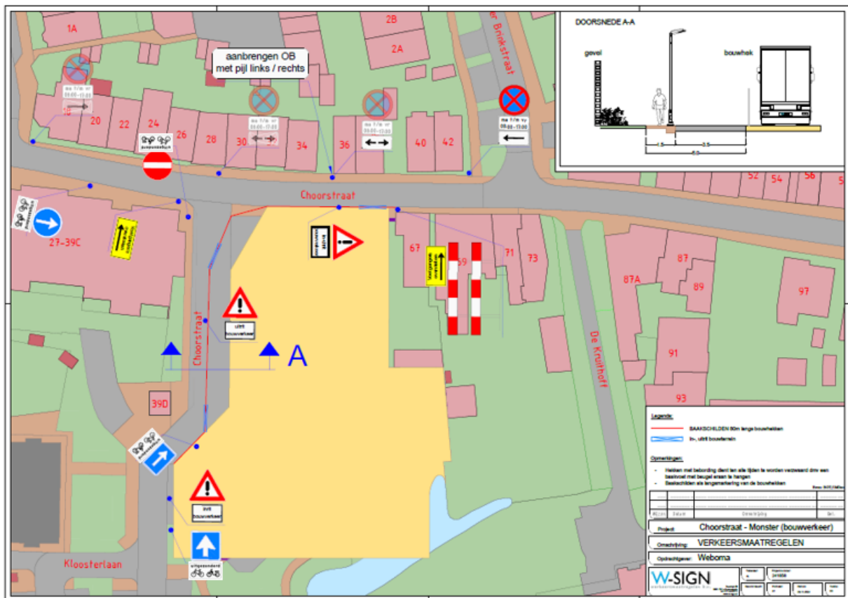
Tekening met kenmerk 241858
