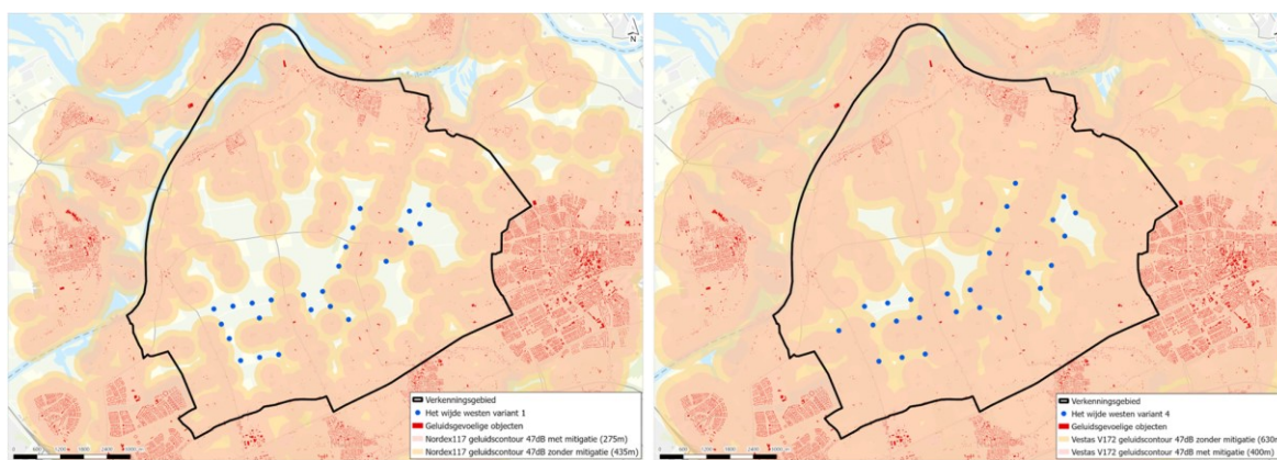
Afbeelding 5.2 De 47 dB L_{den} geluidscontour met en zonder mitigatie (links: variant 1, rechts: variant 4)
