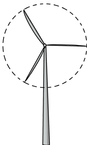
TYPE 2 | VESTAS V172 ashoogte: 175 m rotordiameter: 172 m tiphoogte: 261 m vermogen: 7,2 MW energieopbrengst: 24.000 MWh/jaar
