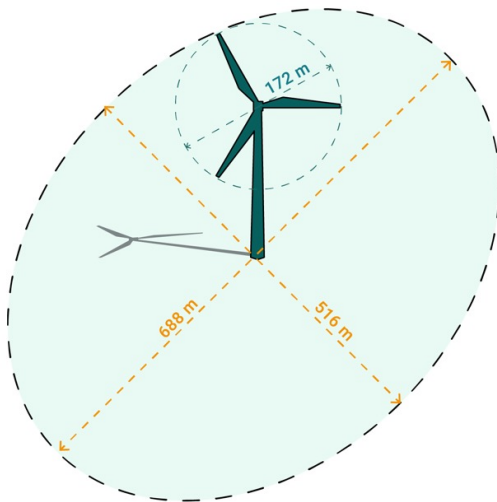
Plaatsingsafstand turbine type 2 (T2)
