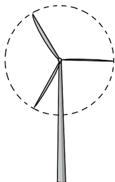
TYPE 1 | NORDEX N117 ashoogte: 134 m rotordiameter: 117 m tiphoogte: 192,5 m vermogen: 3,6 MW energieopbrengst: 12.000 MWh/jaar
