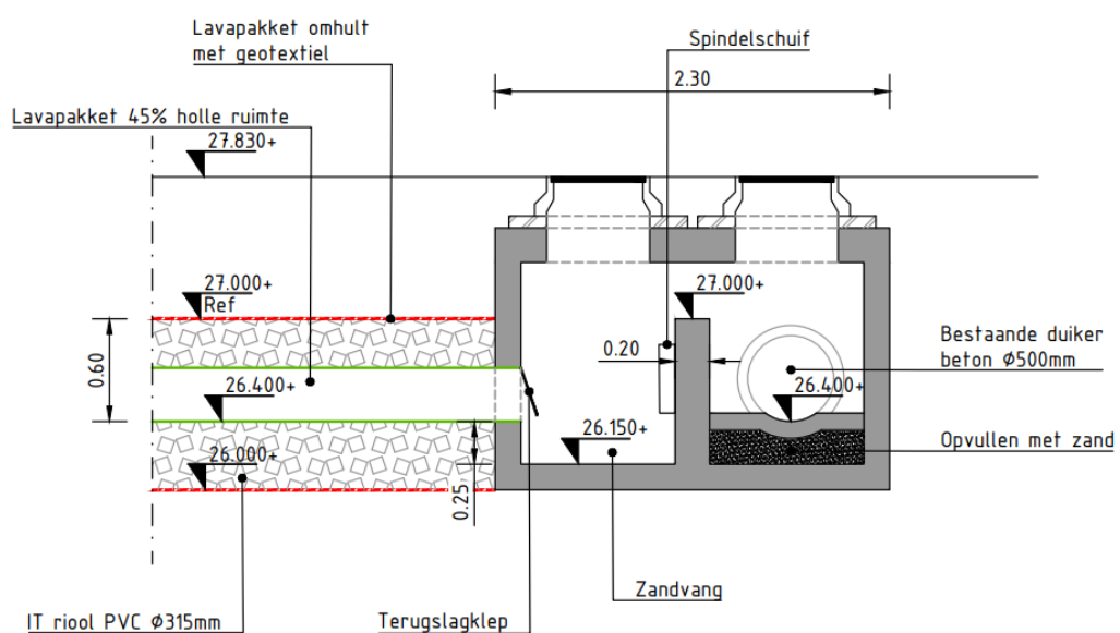
Detail 01: Hondenhokinspectieput met overstort
