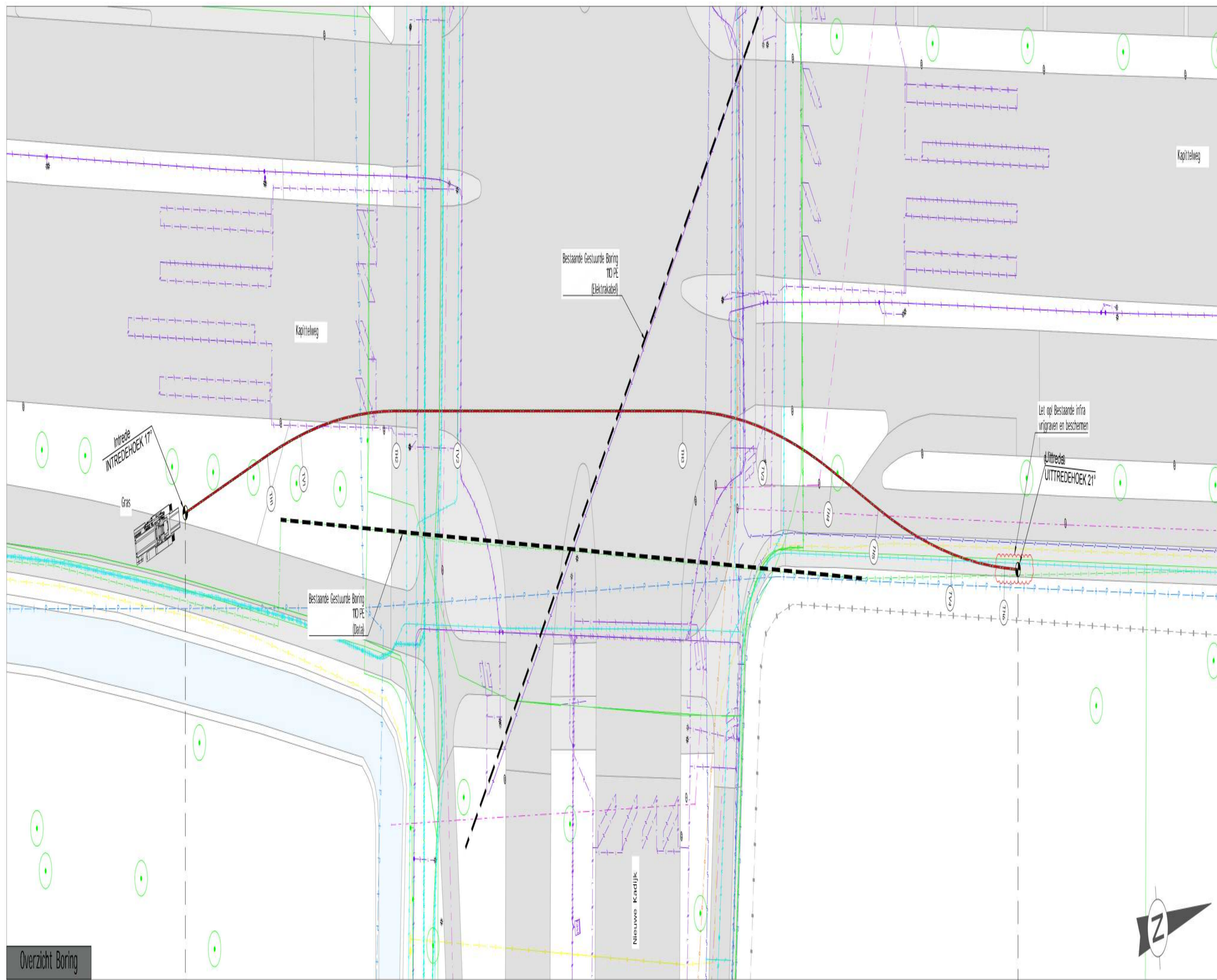
Situatie 1:500
