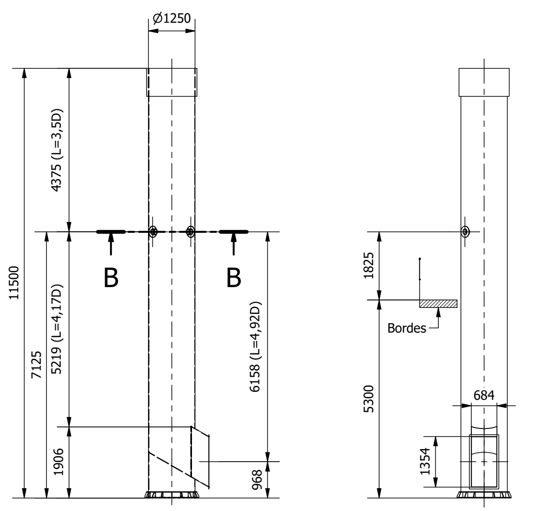
SCHOORSTEEN S-01 ( 1 : 100 )
