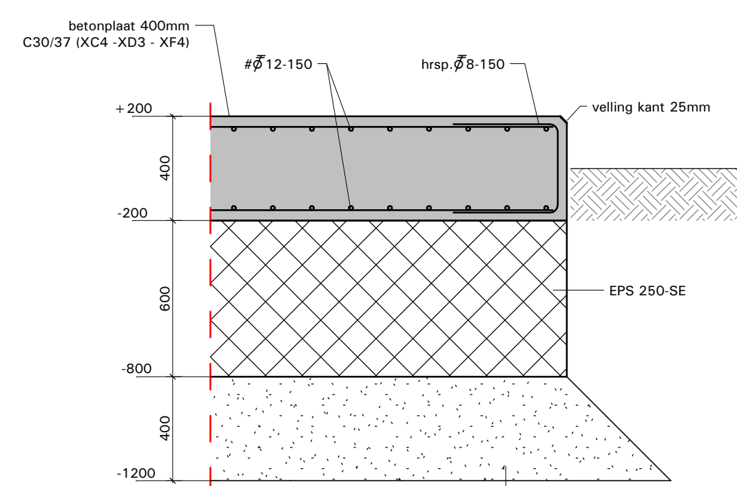
Det. 01 1 : 20
