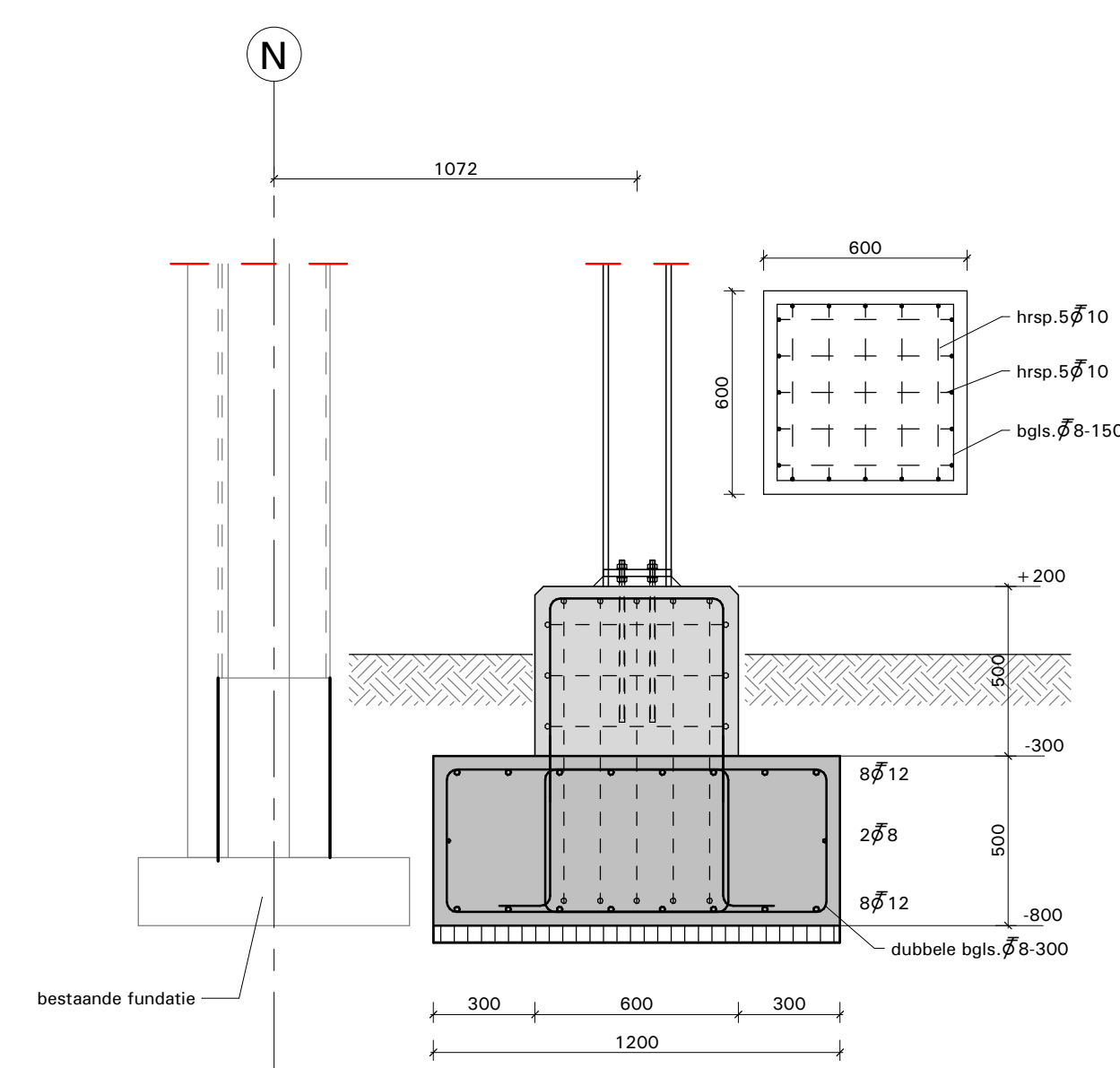
Det. 02 1 : 20
