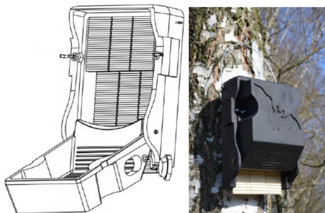
Afbeelding 7: SCHWEGLER vleermuiskast 3FF (bron: www.waveka.nl )
