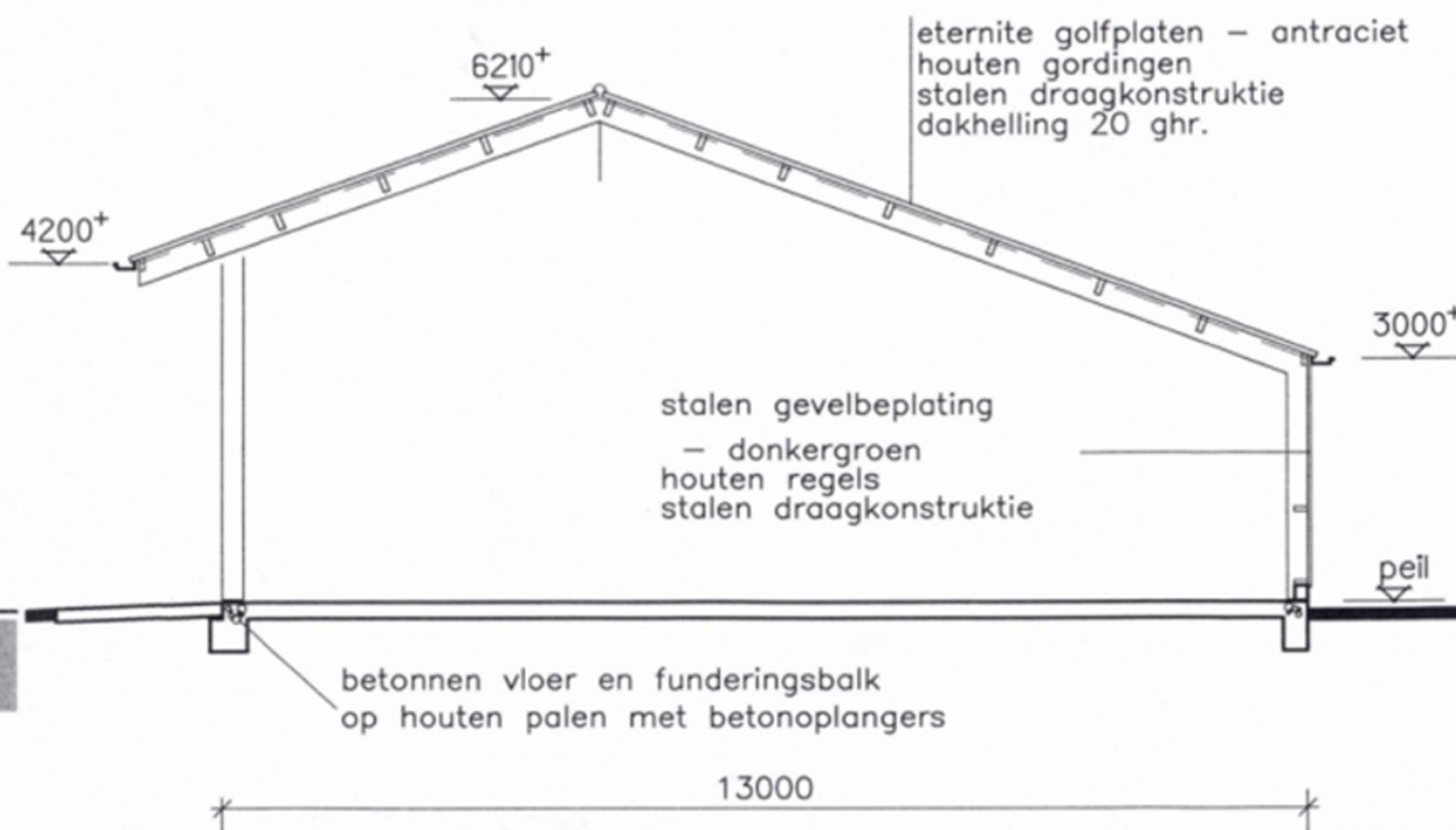
doorsnede
