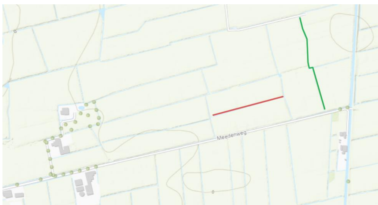
Figuur 1: Locatie van activiteiten. De rode lijn geeft reeds gedempte watergang weer. De groene lijnen geven te verbreden watergangen weer ter compensatie van de verloren gegane waterbergingscapaciteit.
