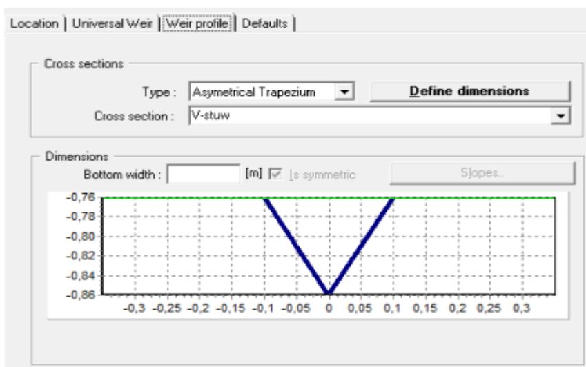
Figuur 2: voorgestelde stuwprofiel uit aanvullingsdocument van 10 september 2024.
