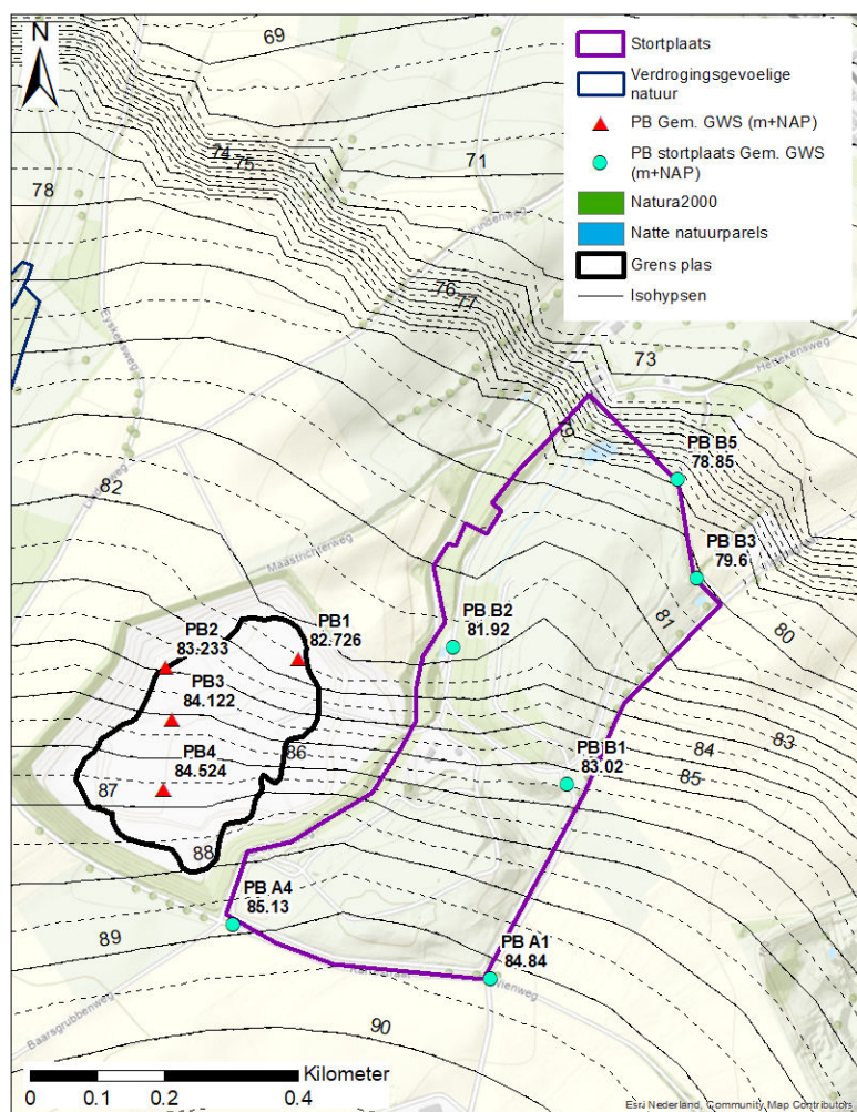
Figuur 4-1 Berekende grondwaterstand Ibrahim V22 Z (isohypsen) en gemiddelde grondwaterstanden in de groeve en rond de vuilstort, ongekalibreerd
