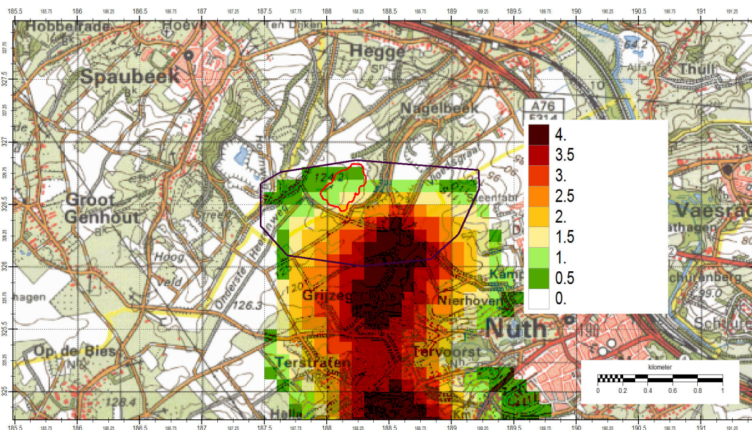
Figuur 4-2 Dikte en locatie van de bruinkoollaag in het model. De zwarte polygoon geeft het gebied aan waarin de weerstand van de bruinkool verlaagd is (tenzij de weerstand al kleiner was dan 300 dagen), de rode polygoon de plas.
