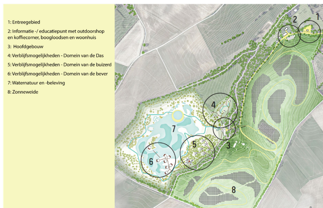
Figuur 1-2: Inrichting plangebied (Bron: Masterplan Groevepark Schinnen-Spaubeek Silt d.d. 20210409.
