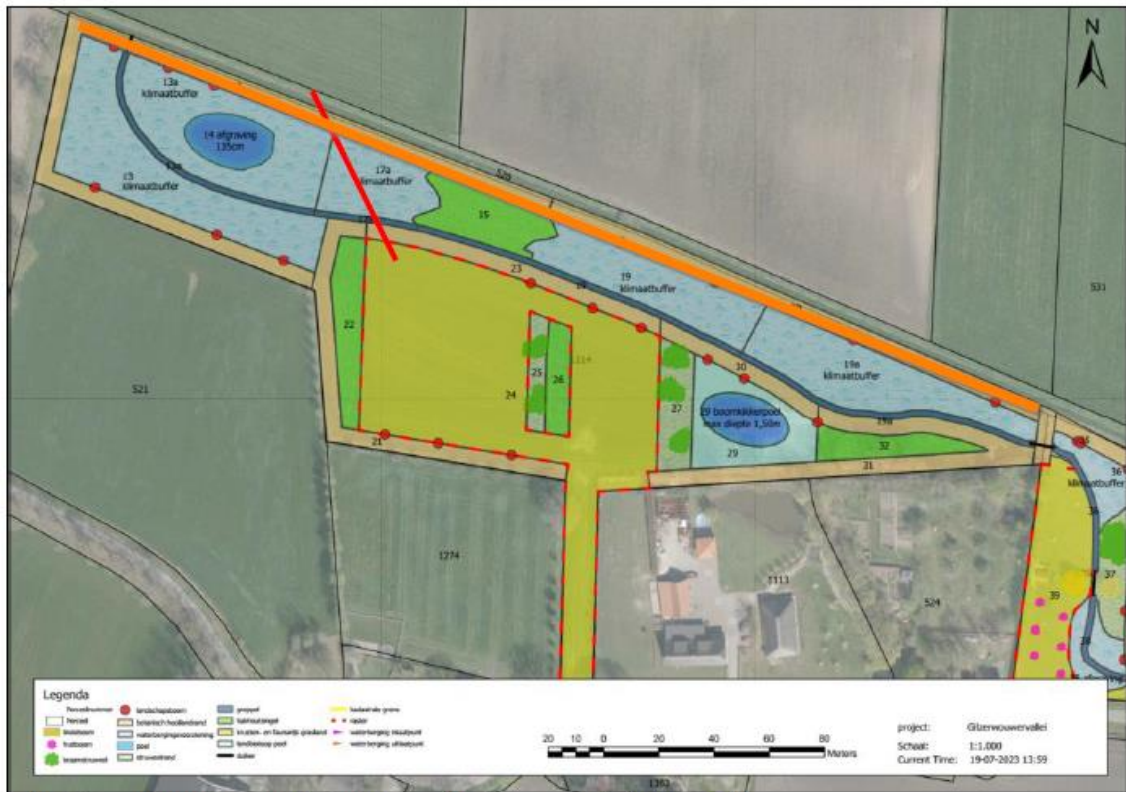
Afbeelding 3; Boven aanzicht, ontwerp (Brabants Landschap 2024)
