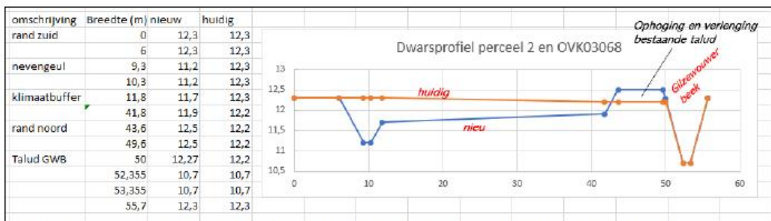
Afbeelding 4; Dwarsdoorsnede, indicatief huidig talud en nieuwe natuurvriendelijke oever.
