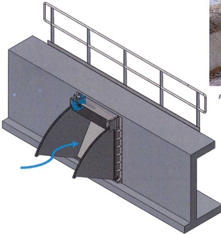
Figuur 4, principe tekening nieuwe stuw met stroomrichting van het water
