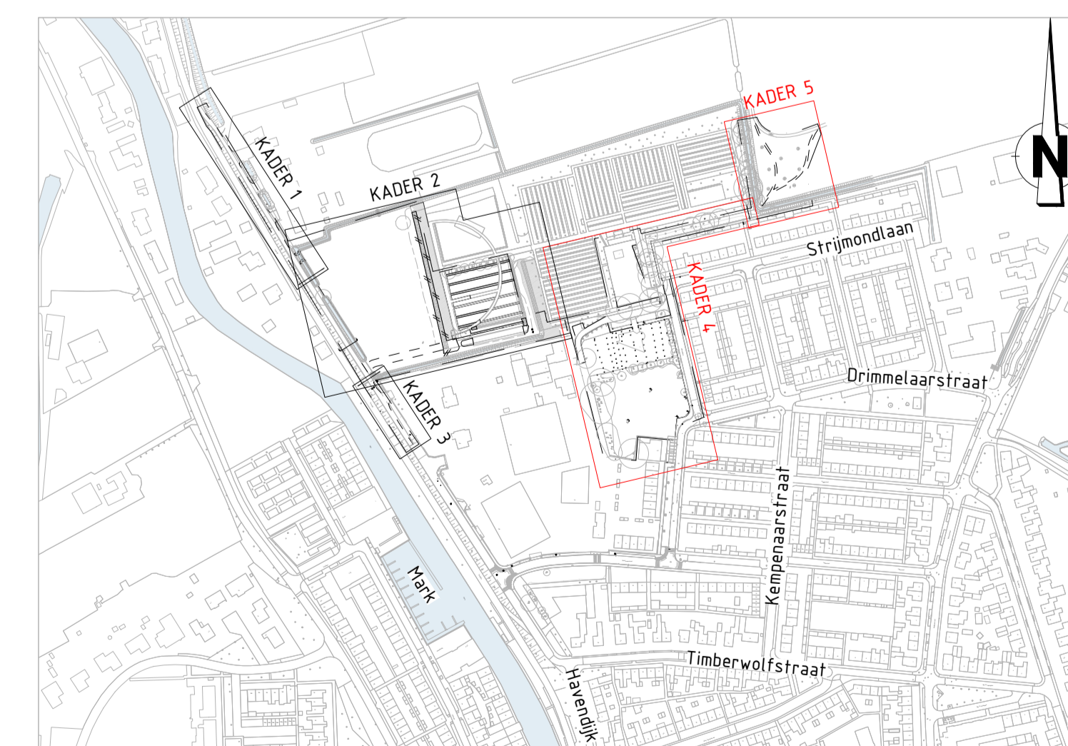
Situatieoverzicht SCHAAL 1 : 4000
