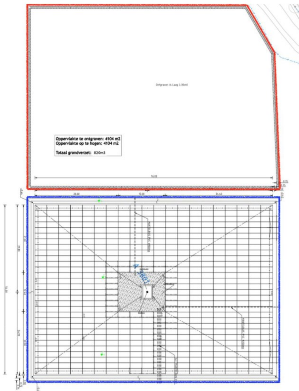
Figuur 4: Af te graven terrein (rood) en op te hogen terrein (blauw)
