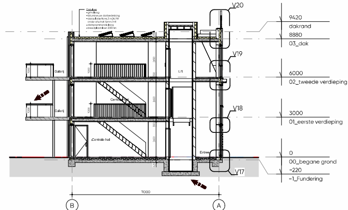
Doorsnede E-E
