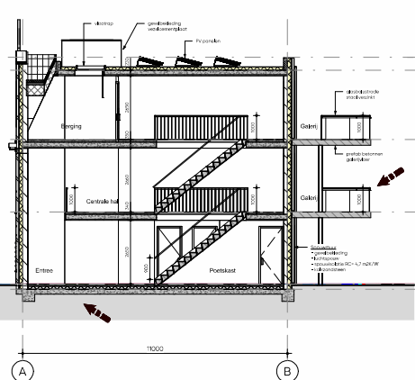
Doorsnede D-D
