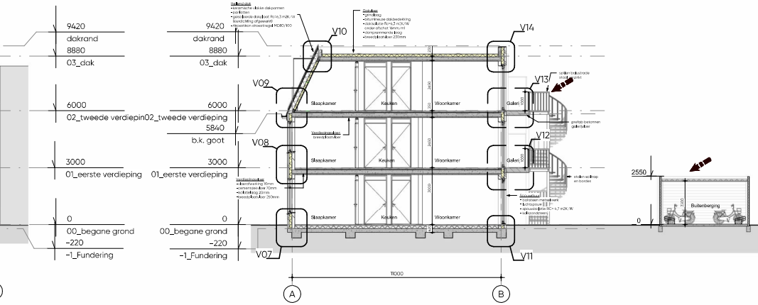
Doorsnede B-B
