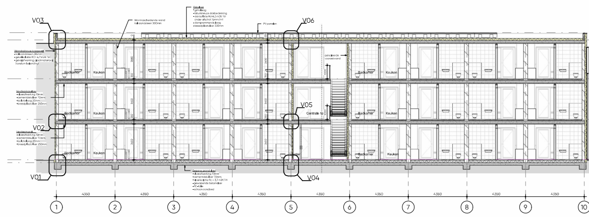
Doorsnede A-A
