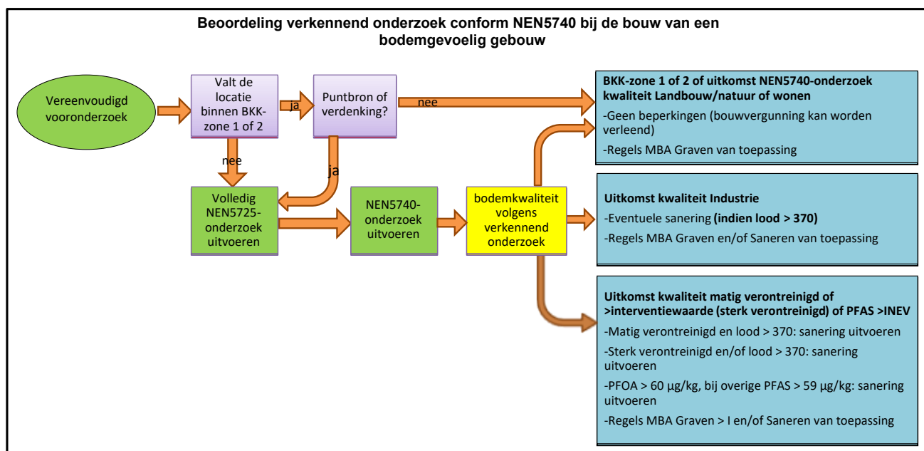
Figuur 8.1 Schema beoordeling noodzaak verkennend onderzoek conform NEN5740 bij de bouw van een bodemgevoelig gebouw
