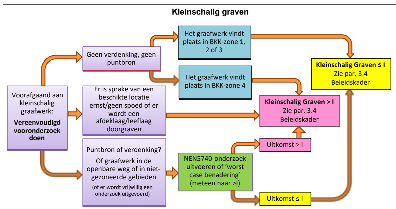
Figuur 3.2 Schematisch overzicht Kleinschalig graven
